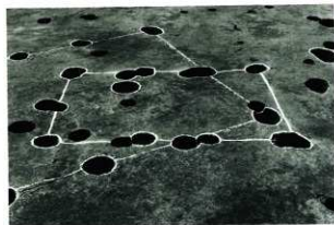
沖田 I 遺跡第 4 号掘立柱建物跡
