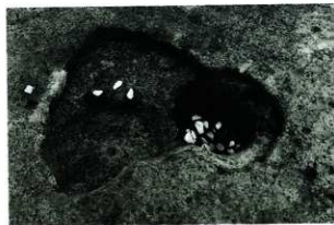
沖田 I 遺跡第 11 号土曜遺物出土状況
