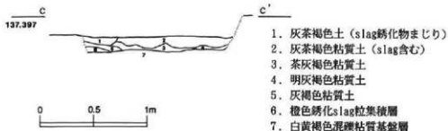
第19図 炉床断面図
