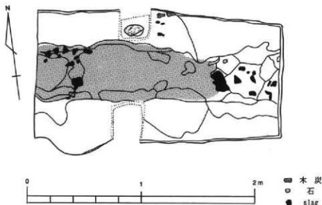
第42図 2号炉実測図
