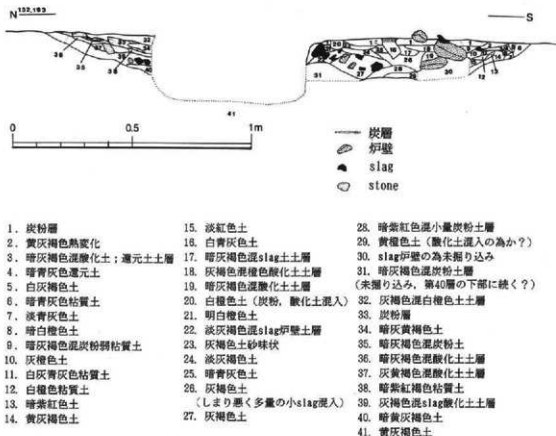
第53図 1号炉断面図
