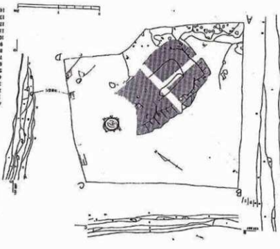
第1回 測量図
