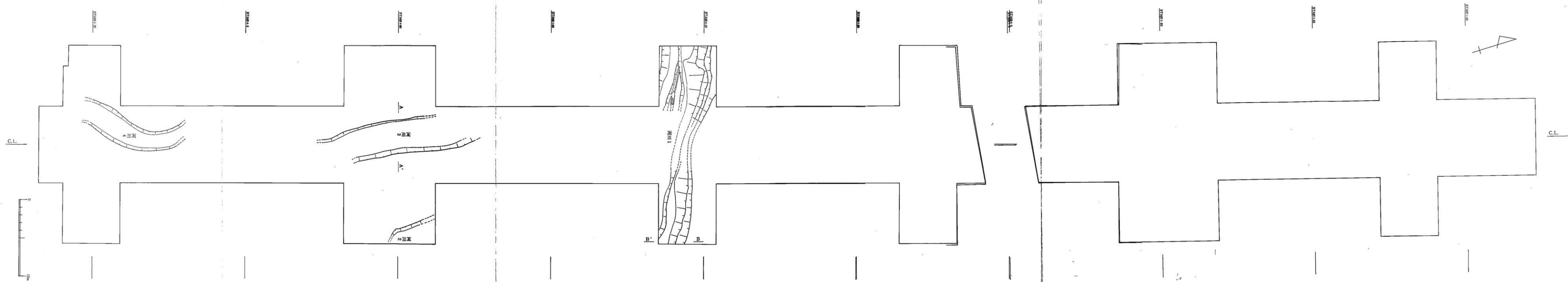
付图1 魏文晚明遗榭面平面图 S=1/200
