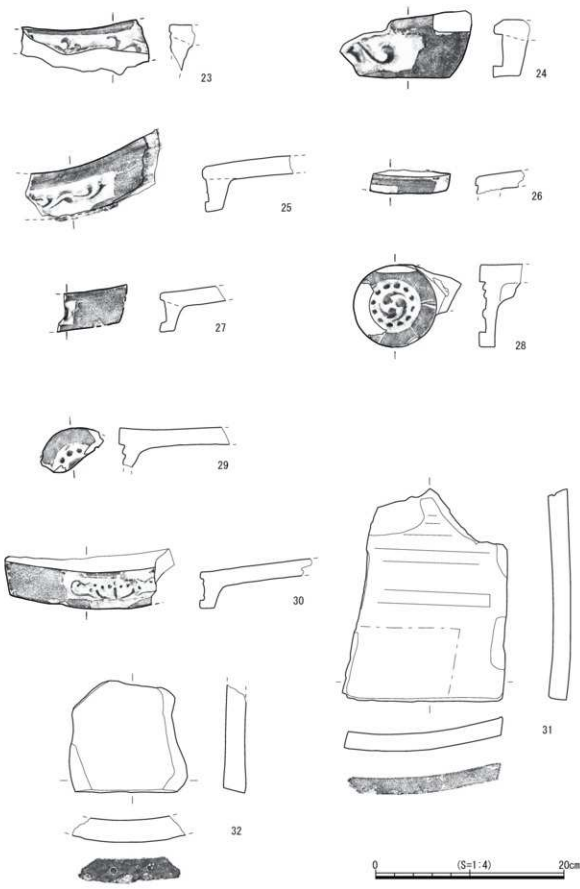
图 28 令和元年度出土遺物実測図 3(瓦)
