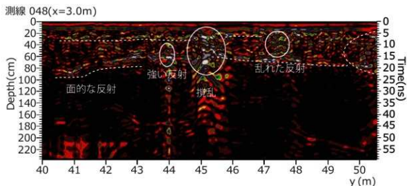
図 11 側線 048 プロファイル図 (40 ~ 50m 付近)
