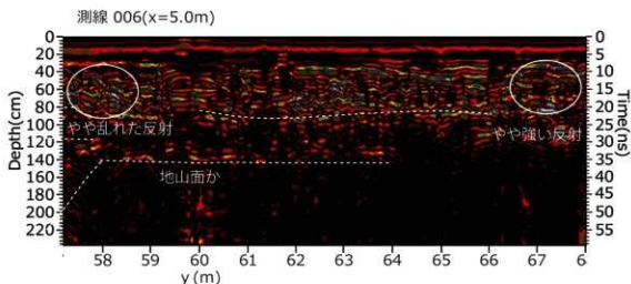
図 12 側線 006 プロファイル図 (58 ~ 64m 付近)
