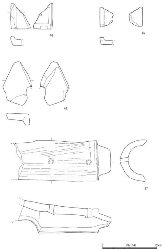
图 31 令和元年度出土物実測图 6 (瓦)
