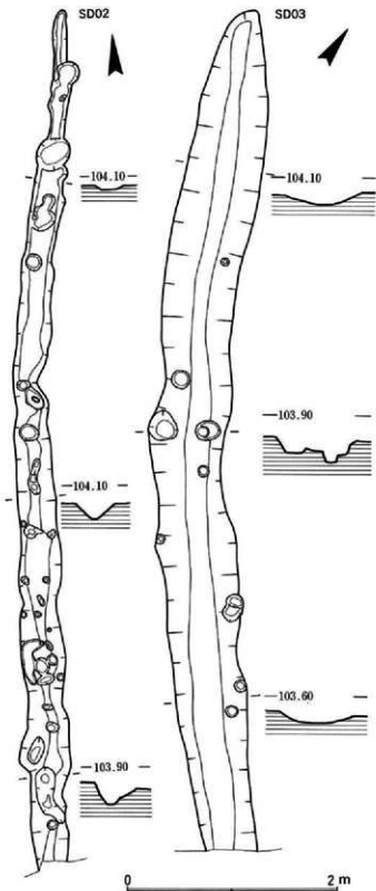
第9図 南区溝実測図
