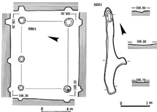
第4図 北区掘立柱建物・溝実測図
