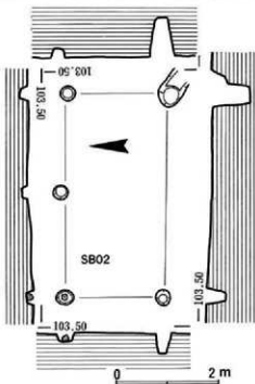
第7図 南区掘立柱建物実測図
