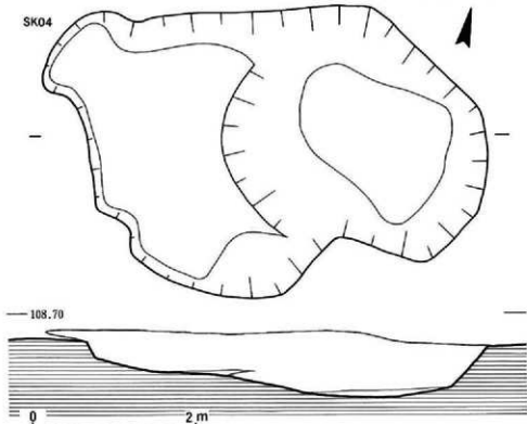
第6図 北区土坑実測図(2)
