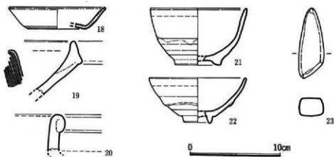
第12図 遺物実測図(2)
