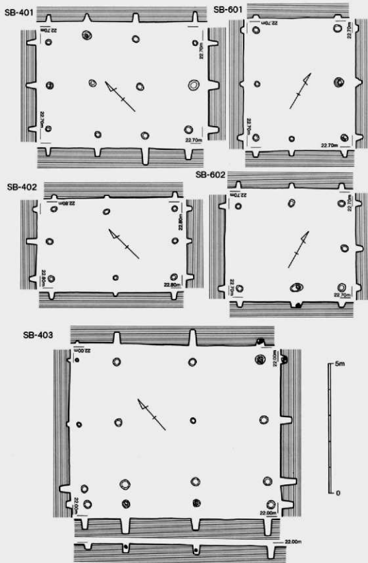
第10图 掘立柱建物実測(図3)
