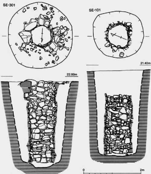
第11図 井戸実測図(1)
