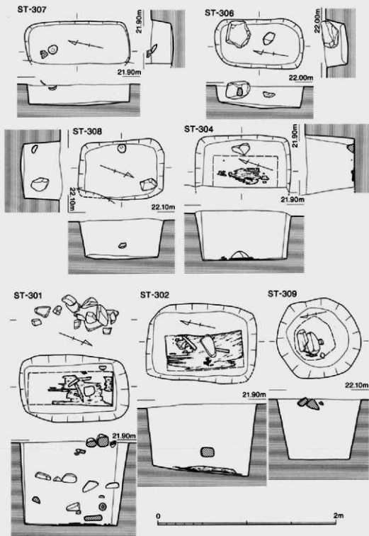
第17图 III地区墓穴测图
