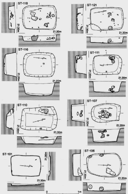
第14图 I地区墓实测图(1)
