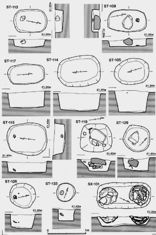
第16图 I地区墓·埋葬遺構実測図
