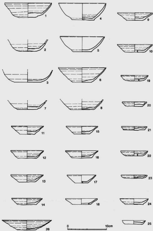
第20图 出土土器夹测图(1)
