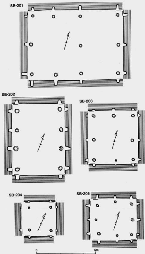
第8圖 掘立柱建物実測(源1) H=21.50m
