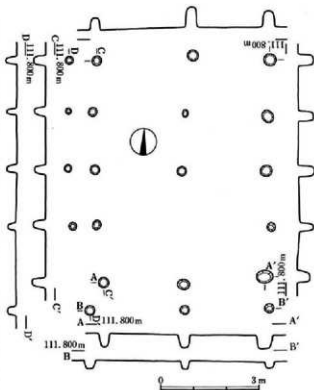
△第10図 掘立柱建物跡（B-4）実測図
