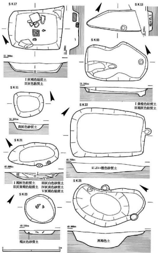
第10図 土坑実測図
