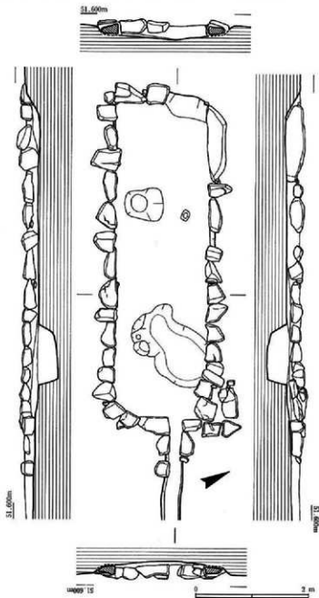
第6図 S F02実測図
