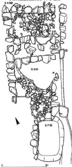
第7図 SF03、SX01・02実測図
