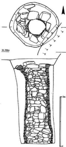
第8図 SE01実測図
