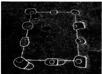
第53号掘立柱建物跡
