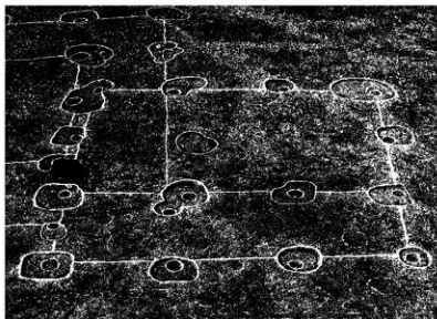
第57号独立柱建物跡
