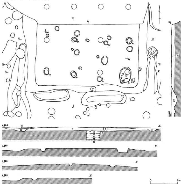
第573図 第1号建物地業跡
