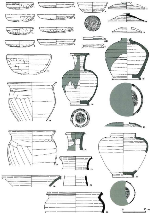
第352图 第203号住居跡出土遺物
