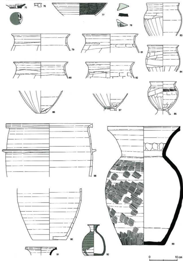
第374图 第217号住居跡出土遺物(3)
