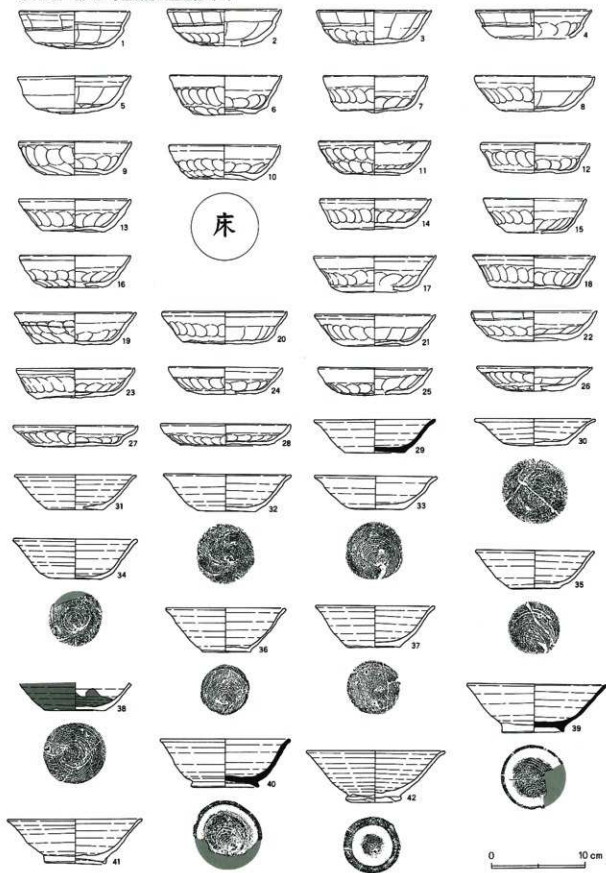
第331图 第197号住居跡出土遺物(1)
