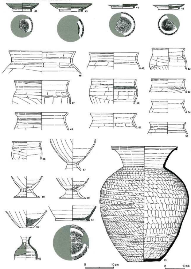
第348图 第202号住居跡出土遺物(2)
