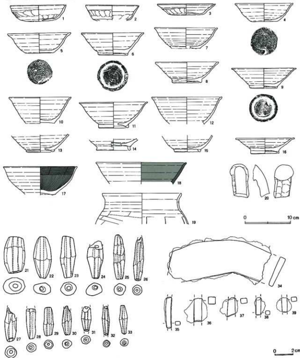
第336図 第198号住居跡出土遺物
