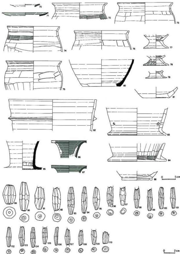
第333图 第197号住居跡出土遺物(3)
