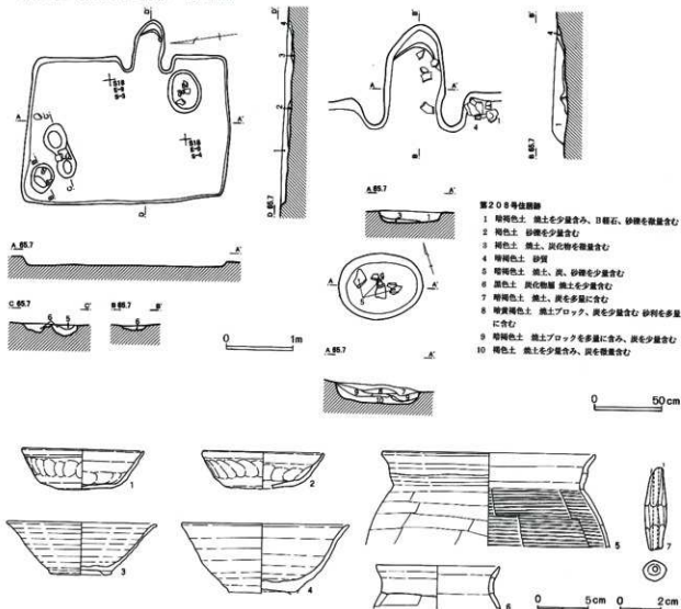
第360図 第208号住居跡・出土遺物
