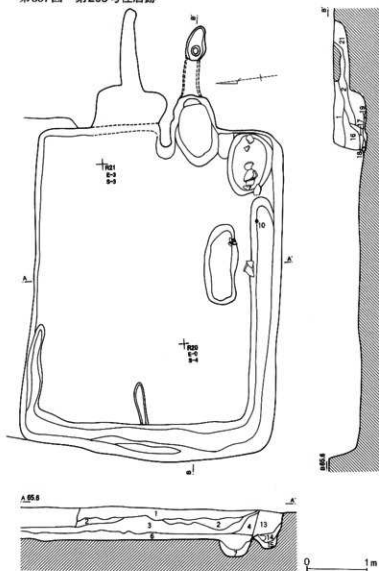
第357図 第205号住居跡
