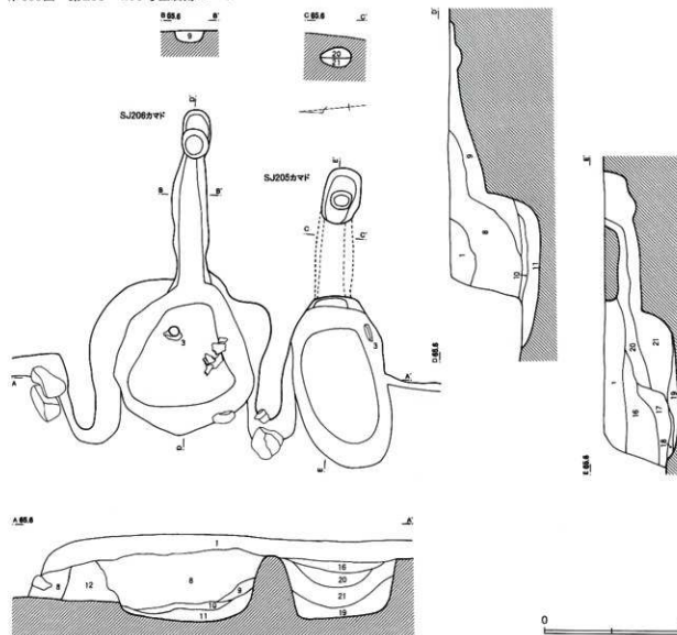
第356図 第205・206号住居跡カマド
