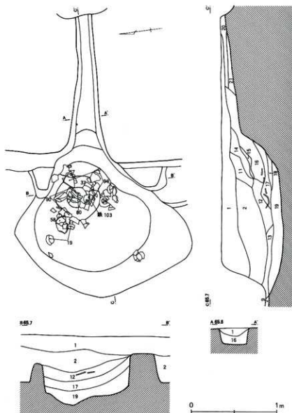
第370図 第217号住居跡カマド
