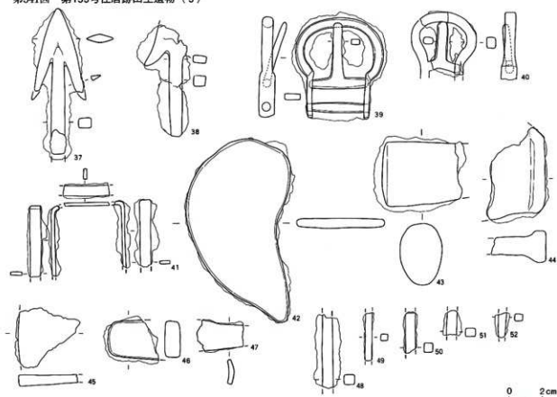
第341図 第199号住居跡出土遺物(3)
