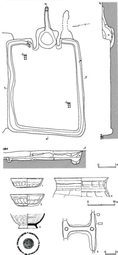
第355図 第206号住居跡・出土遺物
