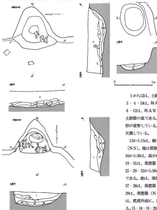
第345図 第202号住居跡カマド・貯蔵穴
