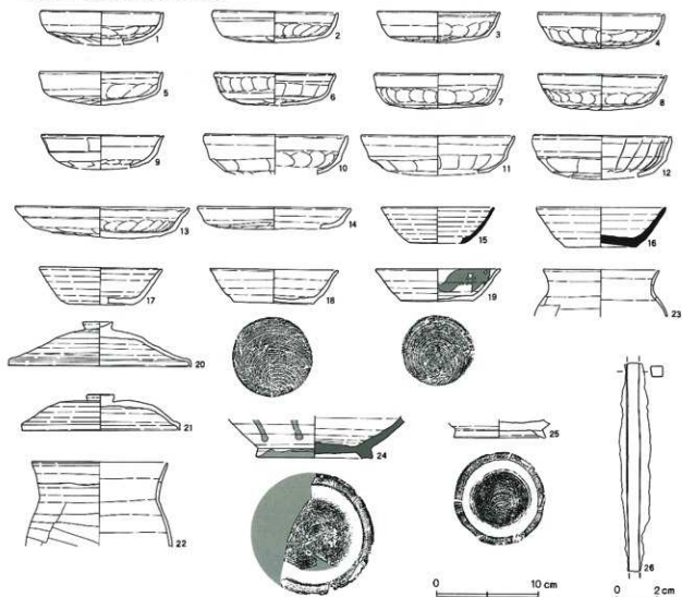
第354図 第204号住居跡出土土遺物
