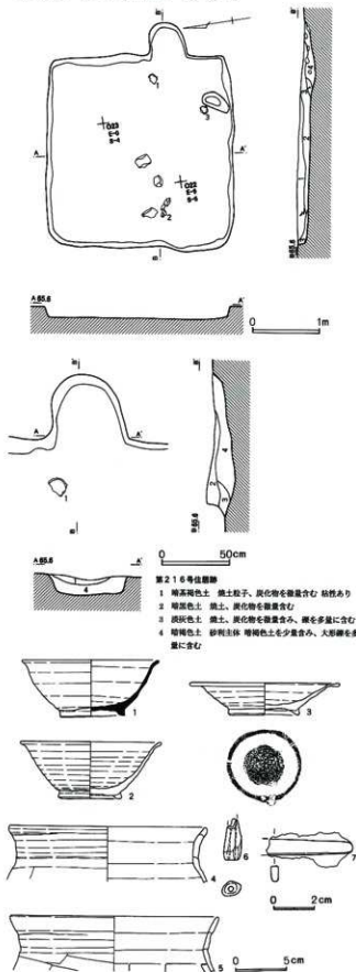
第368図 第216号住居跡・出土遺物
