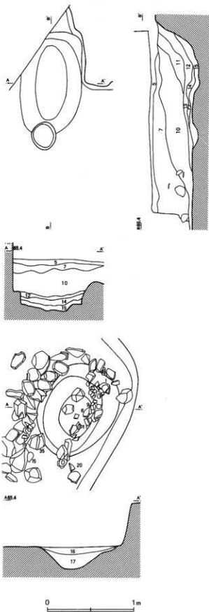
第268図 第155号住居跡カマド・貯蔵穴
