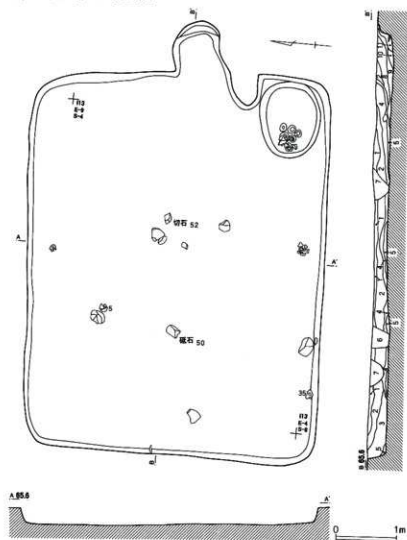
第260図 第152号住居跡
