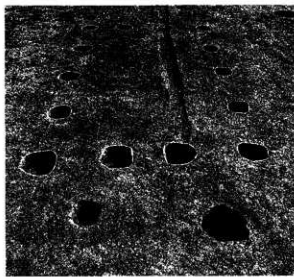
11号掘立柱建物跡
