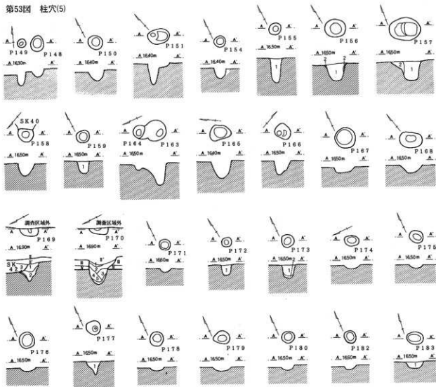
第53図 柱穴(5)
