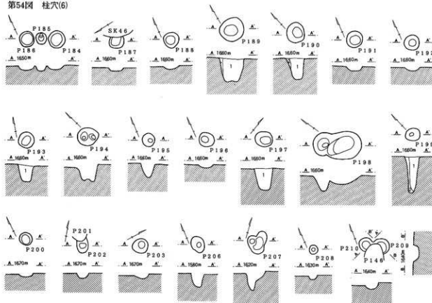
第54図 柱穴(6)
