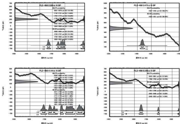
第 12 図 暦年較正年代グラフ
