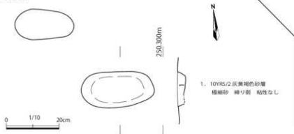
第7図 噴砂及び個別遺構図
