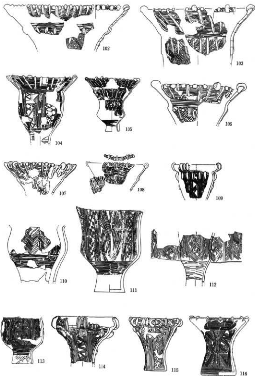
13図 III b 期の土器
