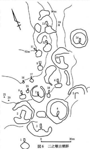
図6 二之塚古墳群
