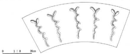
4 図 追貝原出土土器
