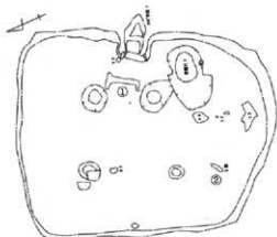
西平井久保田代遺跡3区-8号住居跡
