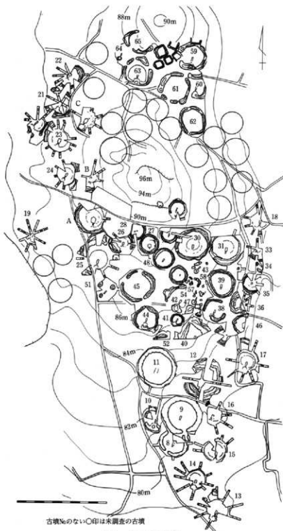
図2 蟹沼東古墳群
