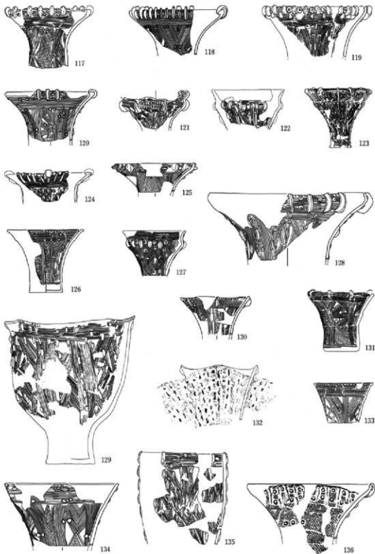
14図 III b期の土器
