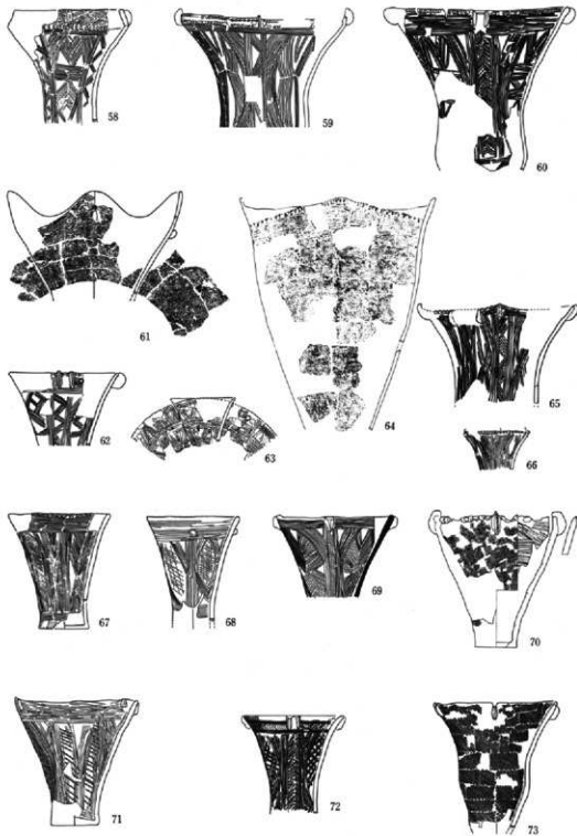
10図 II b 期の土器
