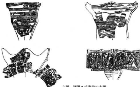
3 図 諸磯 c 式直前の土器
