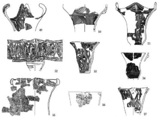
9 図 上段II a 期の土器 下段II b 期の土器
