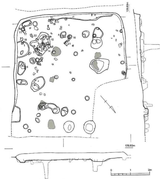
第48図 金山遺跡1次調査区SH10実測図 (1/50)
