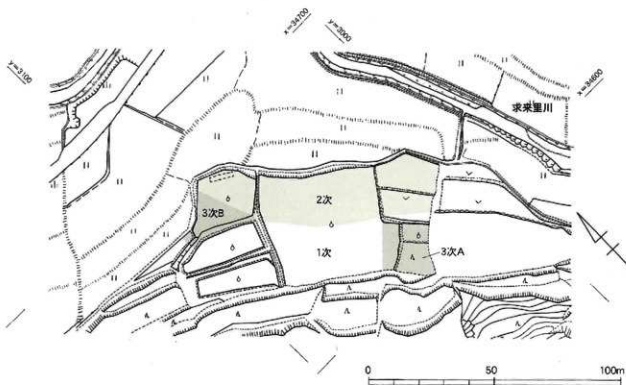
第28図 金田遺跡周辺地形図 (1/1,500)
