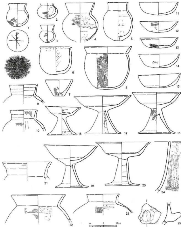
第45図 金田遺跡1次調査区(SH8)出土遺物実測図(1/4)
