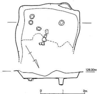
第92図 金田遺跡1次調査区SH34実測図 (1/50)
