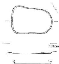
第23図 求来里名里遺跡A区1次調査区 SK100実測図 (1/20)
