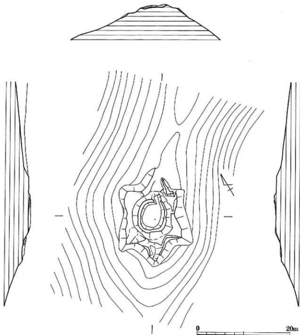
第26図 24号台場実測図
