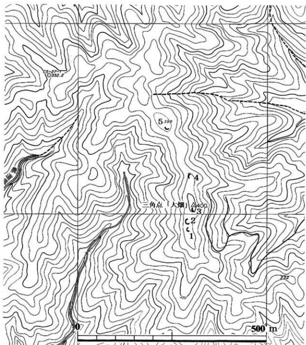
第9図 三角点大畑周辺 (1/5,000図)
