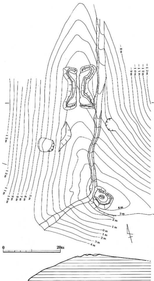
第20図 18号台場(上)・19号台場(下)実測図
