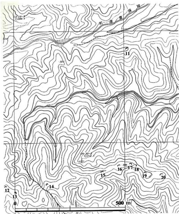
第6図 重岡中学校西側② (1/5,000図)
