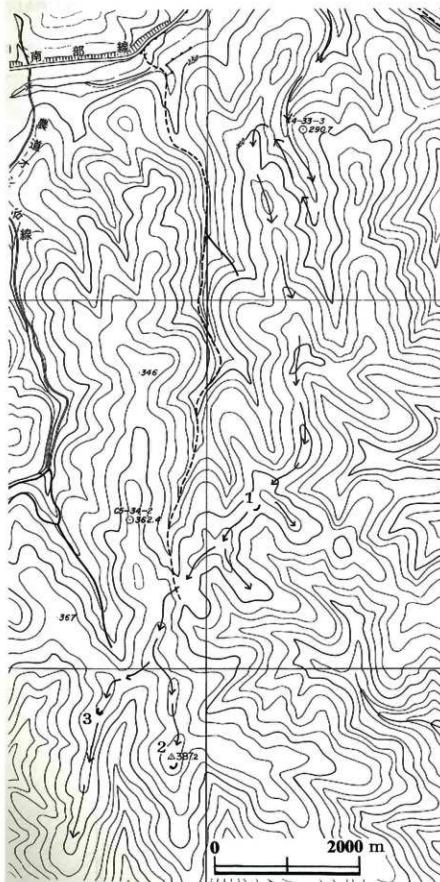
第12図 大原西部（1/5,000図）
