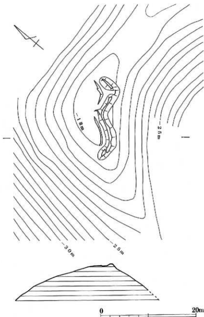
第23回 21号台場実測図
