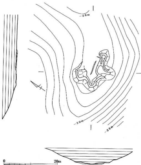
第24図 22号台場実測図
