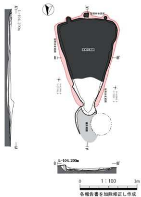
第27図 南玉川Ⅴ遺跡・南玉川Ⅳ遺跡の炭窯跡
