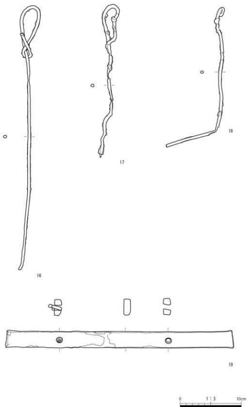
第21図 炭窯跡 SW01 出土遺物 金属製品 (3)
