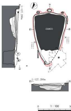
第27図 南玉川Ⅴ遺跡・南玉川Ⅳ遺跡の炭窯跡
