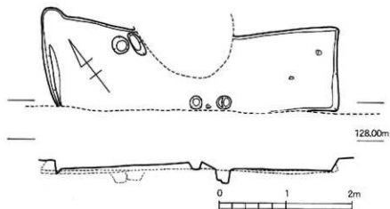
第70図 金田遺跡1次調査区SH21実測図 (1/50)
