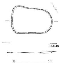
第23図 求来里名里遺跡A区1次調査区 SK100実測図 (1/20)
