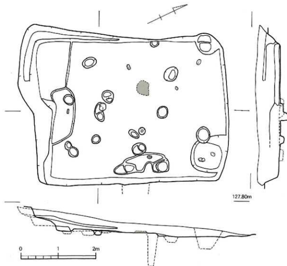
第38図 余田遺跡1次調査区SH5実測図 (1/50)
