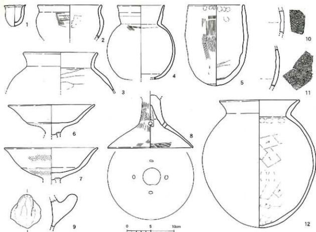
第63图 金山遺跡1次調査区SH17出土遺物実測図 (1/4)
