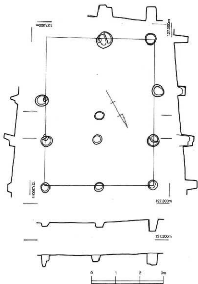
第103图 金田遺跡1次調査区SB3实測図 (1/80)
