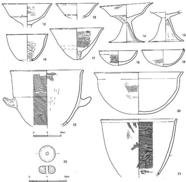
第50図 金田遺跡1次調査区SH10出土遺物実測図 (1～22は1/4、23は1/3)
