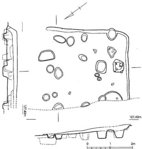
第42図 金田遺跡1次調査区SI17実測図 (1/50)
