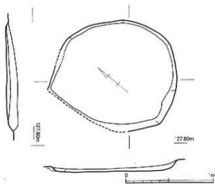
第107図 金田遺跡1次調査区SK2実測図 (1/30)
