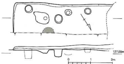
第57図 金田遺跡1次調査区SH14実測図 (1/50)
