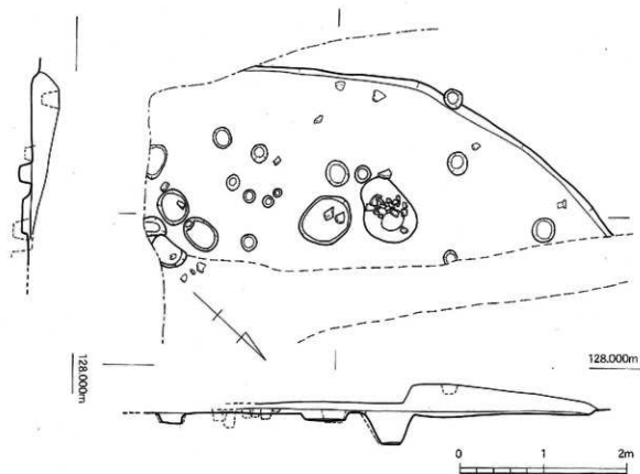
第28図 金田遺跡1次調査区SH1実測図（1/50）
