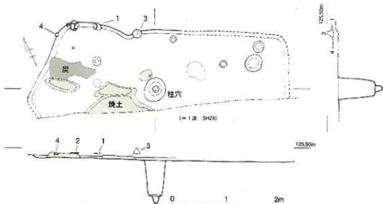
第125図 金田遺跡3次調査区B地区SH209実測図 (1/50)
