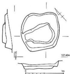
第108図 金田遺跡1次調査区SK3実測図 (1/30)
