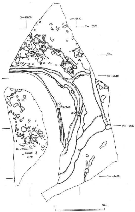
第22图 求来甲各里遗址A区1次调查区遗址配置图 (1/200)
