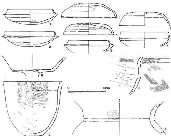
第16图 求来里平岛遗址D区SH6出土遗物实测图 (1/3)
