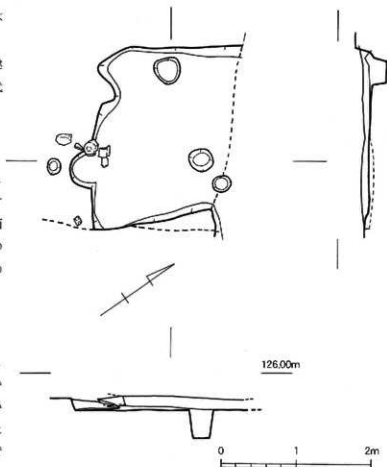
第91図 金田遺跡1次調査区SH33実測図 (1/50)
