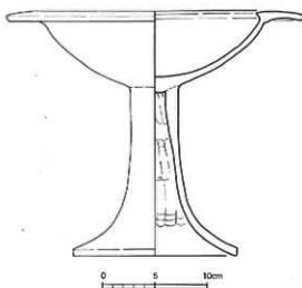
第102图 金田遺跡1次調査区 SB2柱穴2出土遺物実測図 (1/4)
