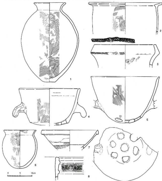
第109図 金山遺跡1次調査区出土遺物実測図 (1/4)
