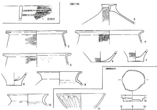
第114図 金口遺跡3次調査区A地区出土遺物実測図 (1/4)
