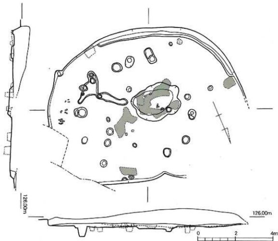
第66図 金山遺跡1次調査区SH19実測図 (1/50)
