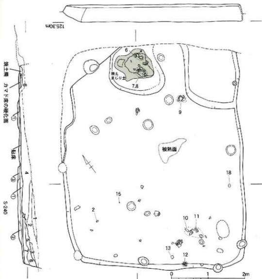
第129図 金田遺跡3次調査区B地区SI1212実測図 (1/50)
