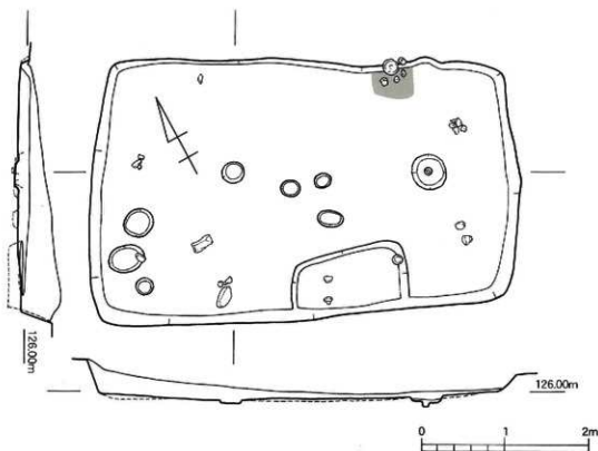
第60図 金田遺跡1次調査区SH16実測図 (1/50)
