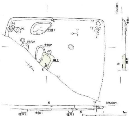
第134図 金田遺跡3次調査区B地区SH1214実測図 (1/50)
