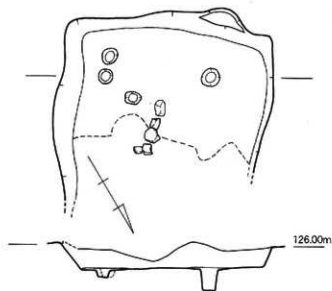
第92図 金田遺跡1次調査区SH34実測図 (1/50)
