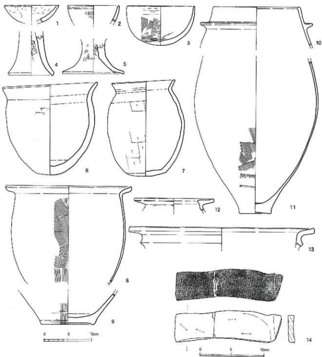
第67図 金田道跡1次調査区SH19出土遺物実測図 (1～13は1/4, 14は1/3)
