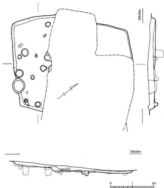
第73図 金州遺跡1次調査KSI123実測図 (1/50)
