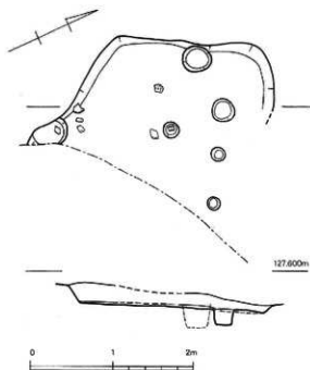
第31図 金田遺跡1次調査区SH2実測図 (1/50)
