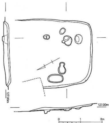
第90図 金田遺跡1次調査区SH32実測図 (1/50)
