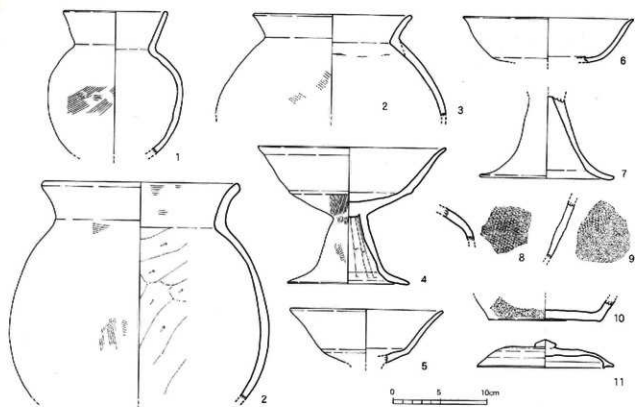
第69図 金田遺跡1次調査区SI120出土遺物実測図 (1/4)
