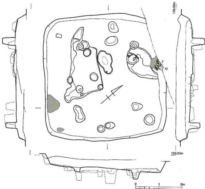
第62図 金田遺跡1次調査区SH17実測図 (1/50)
