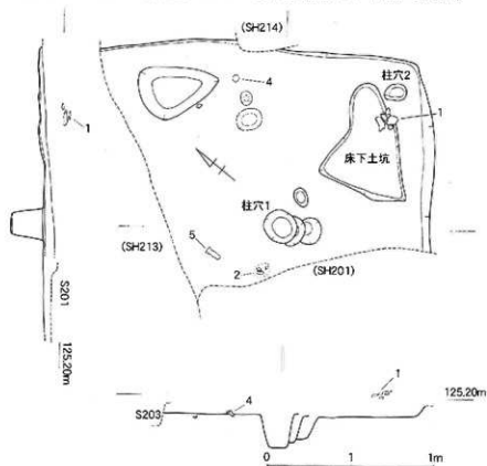
第120図 金田遺跡3次調査K地区SH204実測図 (1/50)
