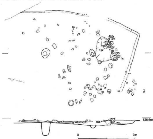
第9図 求来里平島遺跡D区SH4実測図 (1/50)
