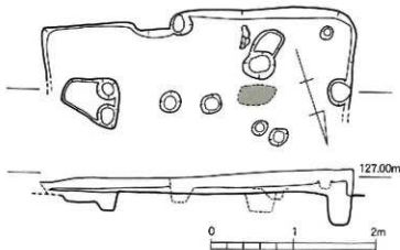
第58図 金田遺跡1次調査区SH15実測図 (1/50)
