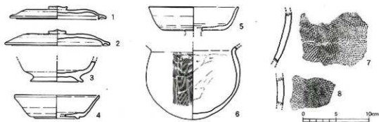
第54図 金田遺跡1次調査区SH12出土遺物実測図 (1/4)
