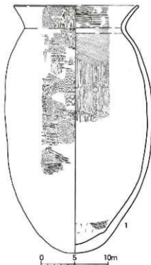
第123図 金田遺跡3次調査区B地区 SH206出土遺物実測図 (1/4)
