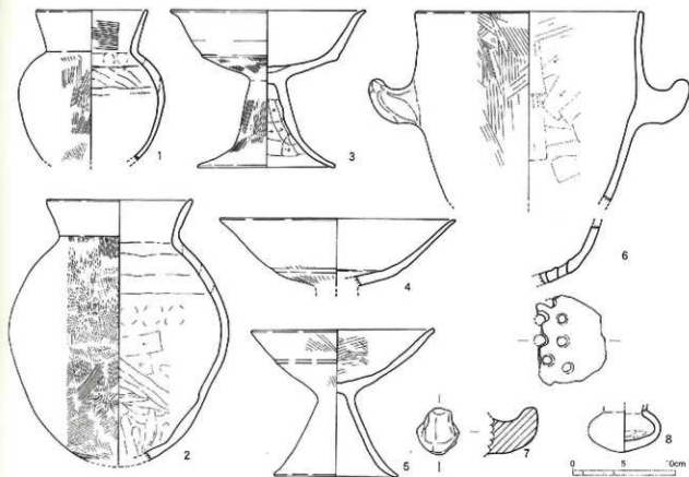
第47图 金山遗址1次调查区SI19出土遗物实测图 (1/4)
