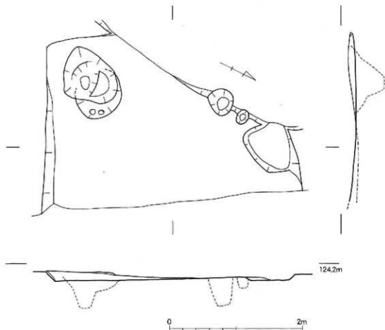
第13図 求東里平島遺跡D×SH5実測図 (1/50)
