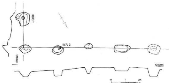
第98図 金田遺跡1次調査区SB2実測図 (1/80)
