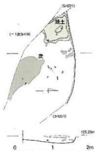
第118図 金田遺跡3次調査区B地区SH202実測図 (1/50)
