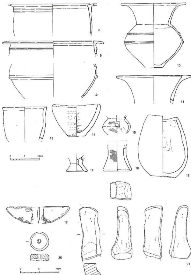
第37图 金山遗址1次調査区SH4出土物実測図 (1/4)
