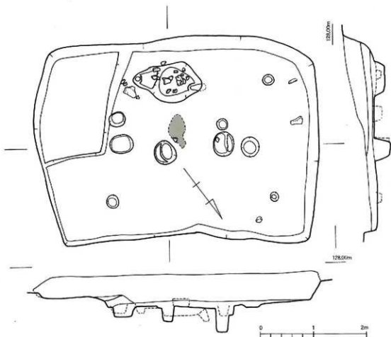
第35図 金田遺跡1次調査区SI14実測図 (1/50)
