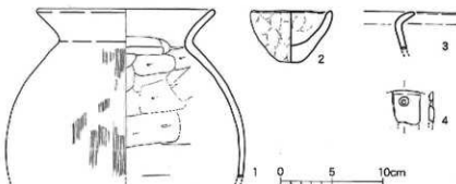
第142図 金田遺跡3次調査区B地区SH255出土遺物実測図 (1/4)
