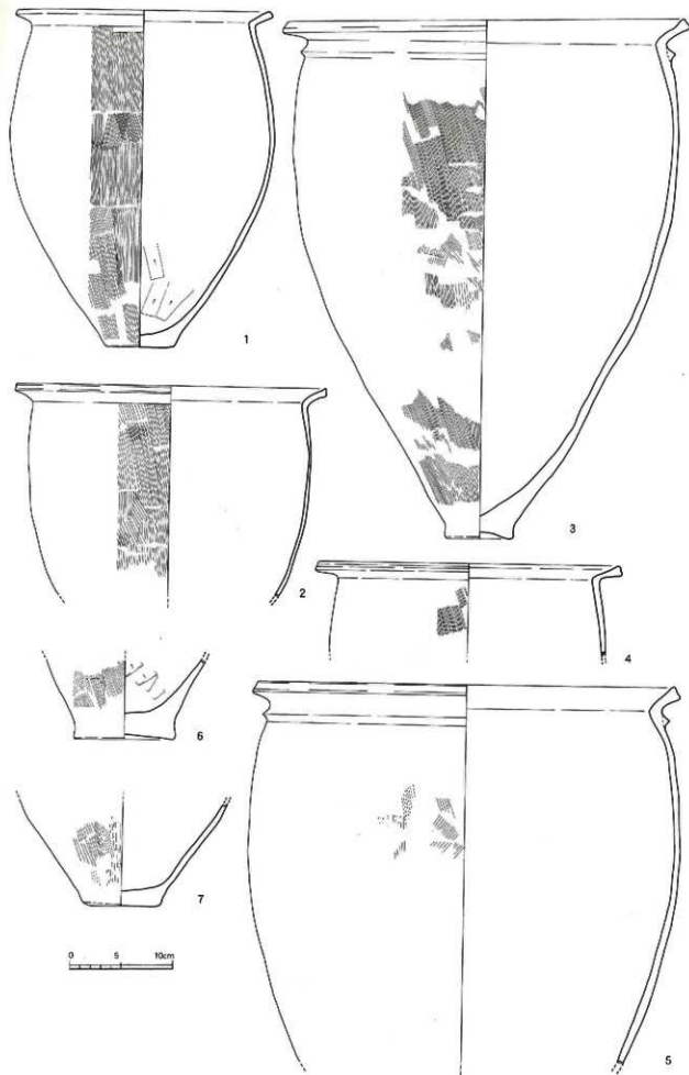
第36圖 金州遺跡1次調査|KSH4出土遺物実測図 (1/4)
