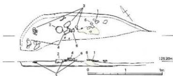
第116図 金田遺跡3次調査区B地区SH201実測図 (1/50)
