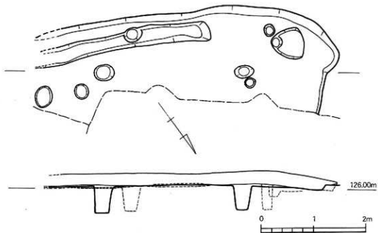
第78図 金山遺跡1次調査区SH26実測図(1/50)
