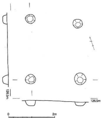
第17图 求来里平岛遗址D区SH7实测图 (1/50)
