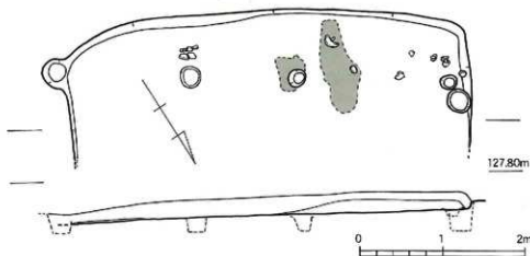
第40図 金田遺跡1次調査区SH6実測図 (1/50)
