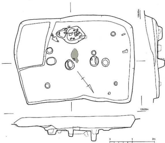
第35図 金田遺跡1次調査区SH4実測図 (1/50)
