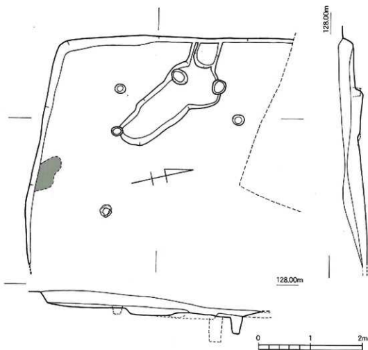
第55図 金田遺跡1次調査区SH13実測図 (1/50)
