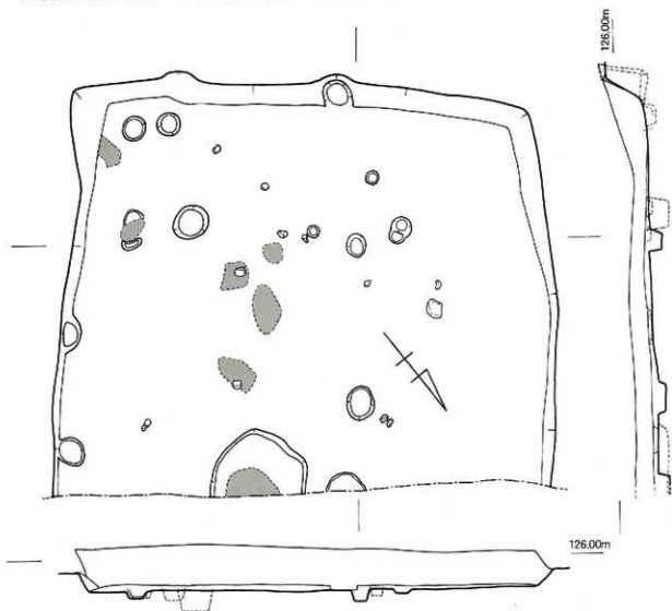
第71図 金田遺跡1次調査区SH22実測図 (1/50)
