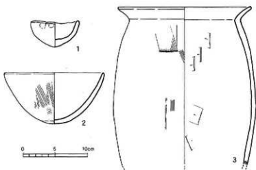
第80図 金山遺跡1次調査区SH127出土遺物実測図 (1/4)
