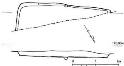
第86図 金田遺跡1次調査区SH130実測図 (1/50)
