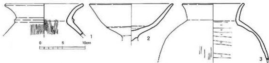
第76回 金田遺跡1次調査区SH23出土遺物実測図 (1/4)
