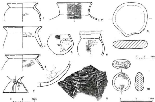
第39図 金田遺跡1次調査区SH5出土遺物実測図（1/4）、石器（1/3、1/6）
