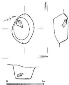
第101图 金田遺跡1次調査区SB2柱穴2実測図 (1/30)
