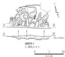
図3-16 ST1遺構図
