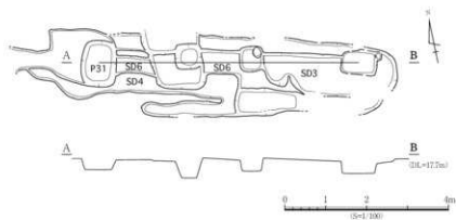
図3-20 SA1遺構図
