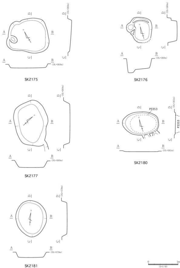
図3-58 SK遺構図
