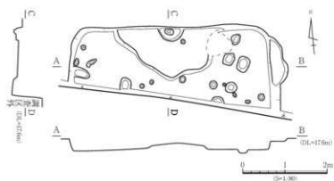
図3-14 ST2024遺構図
