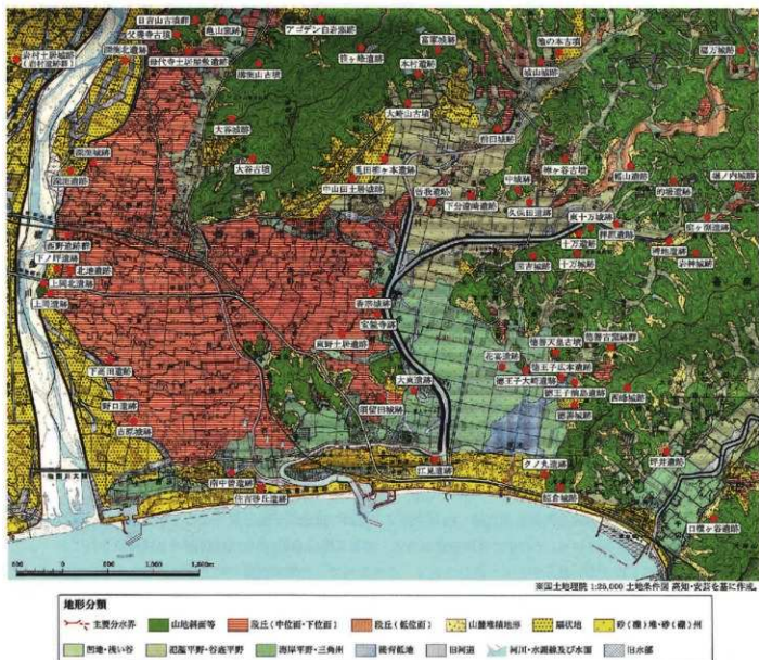
第5図 鹿ヶ洞遺跡周辺の主な遺跡及び地形分類図(S=1/45,000)
