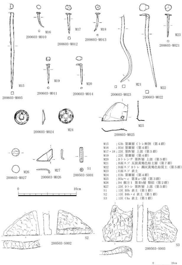
第173図 出土遺物実測図 金属2・石製品 (S=1/2、1/6)
