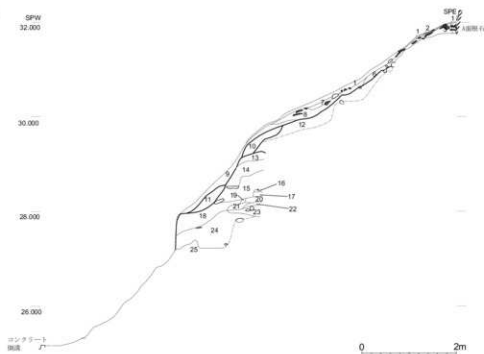
断面 8
