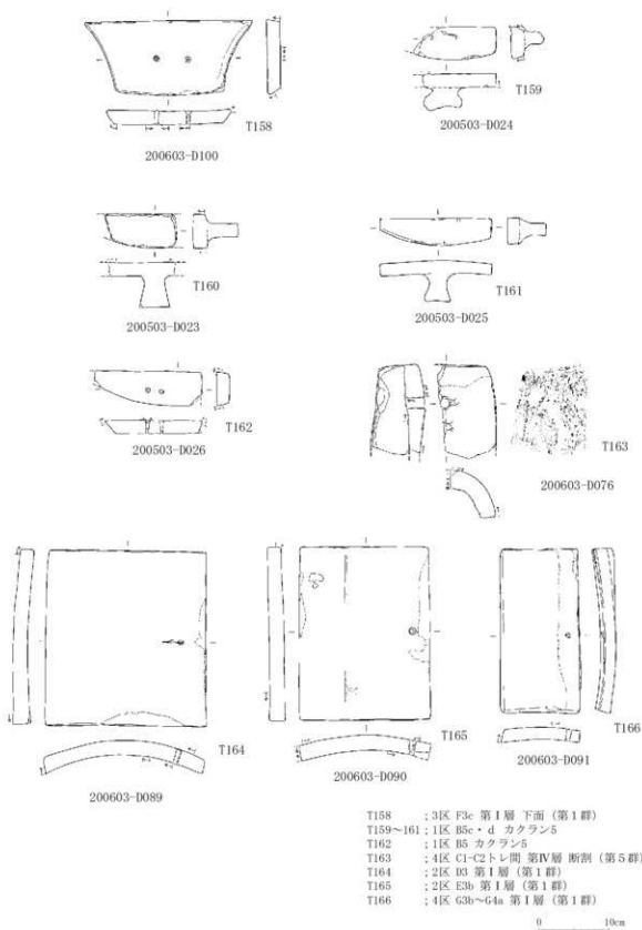
第167図 出土遺物実測図 瓦22 (袖菜, S=1/6)
