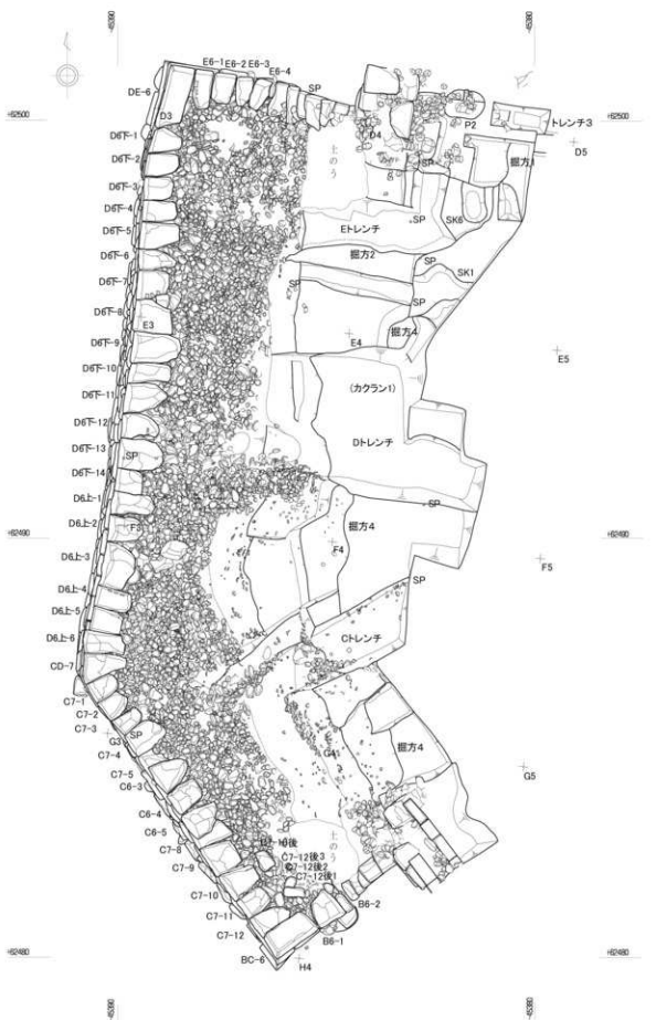
第46図 第10段平面図 (S=1/100)
