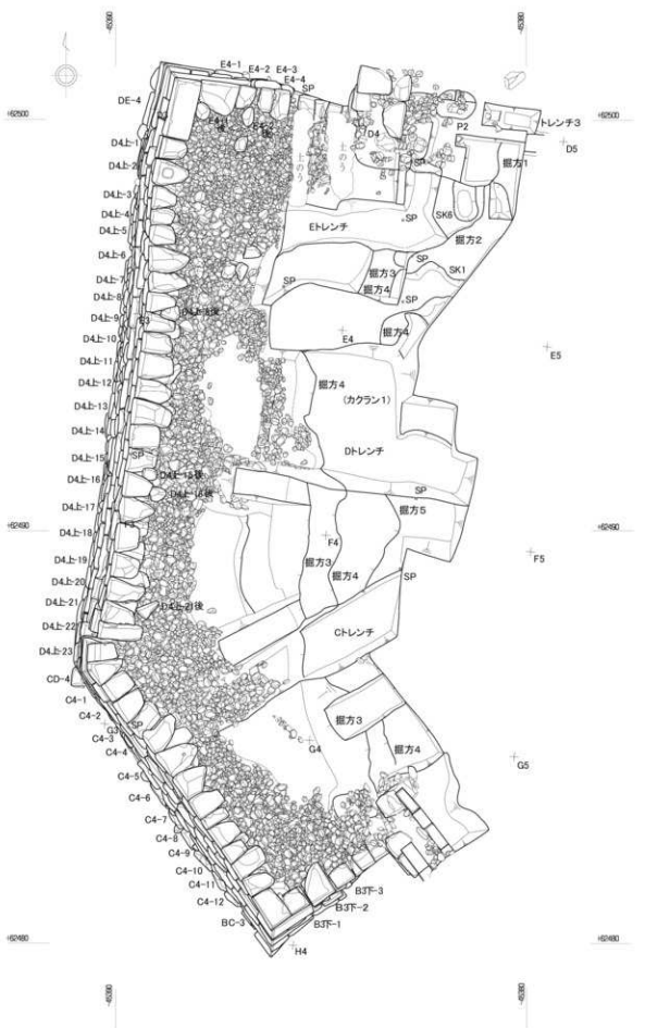
第36図 第6段平面図 (S=1/100)
