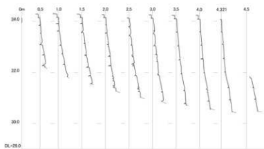
玉泉院丸南西石垣 解体修復後 断面図(垂直) (E面)
