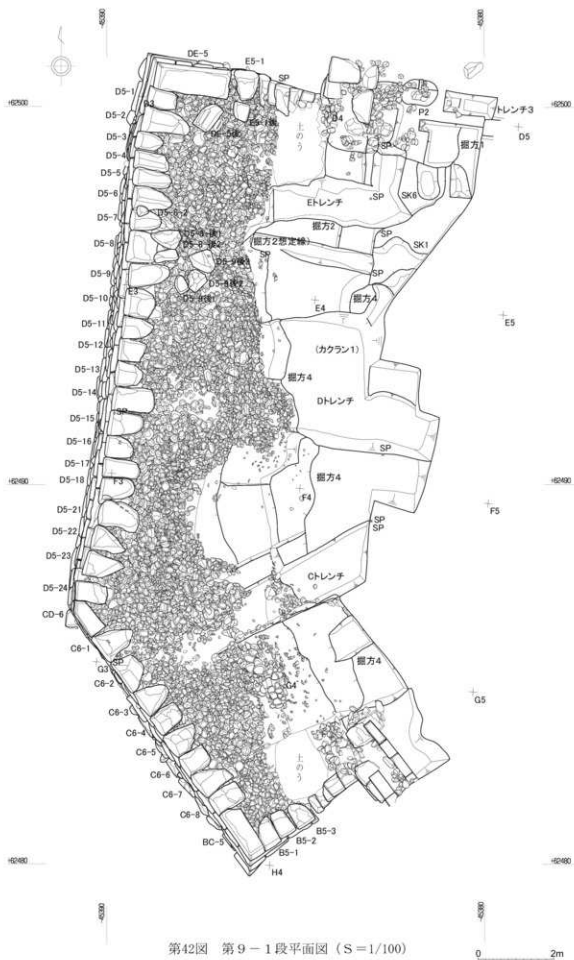
第42図 第9-1段平面図 (S=1/100)
