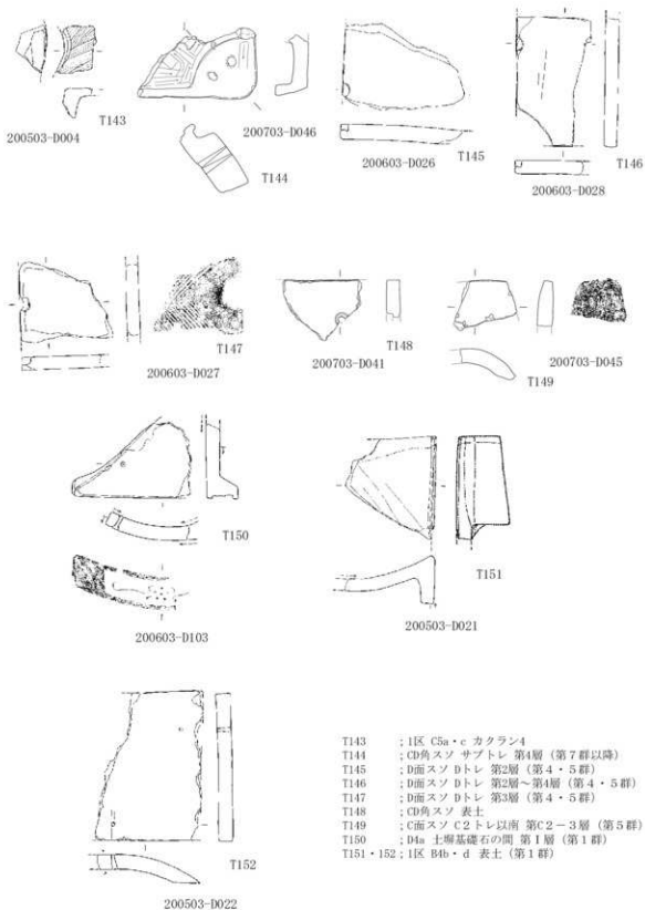
第165図 出土遺物実測図 瓦20 (いぶし・釉, S=1/6)
