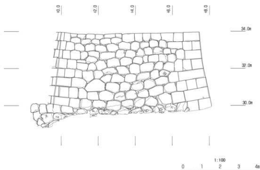
第1图 石垣立面图1
