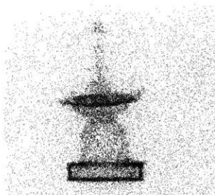
銀製小型宝塔 \gamma 線写真
