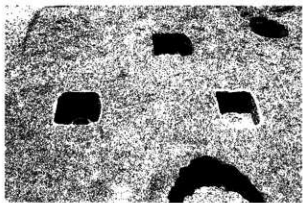
第01号掘立柱建物跡
