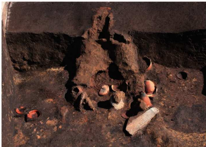
1 46号竪穴建物カマド遺物出土状況(西より)
