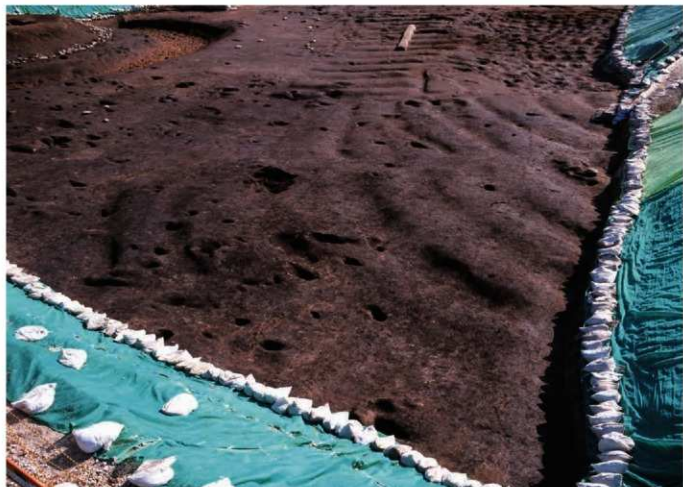
5 屋敷地外畠6・8～10・13号畠(空撮、手前西)
