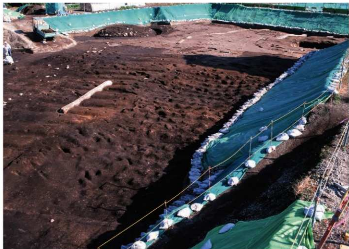
1 11号畝完掘状況(北東より)
