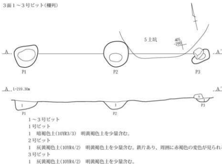
第11図 3面1～3号ピット(柵列)平面図、4号ピット平面図・土層断面図
