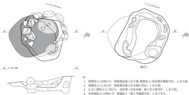
第6図 2面1号坑 4 平面図・掘方平面図・土層断面図
