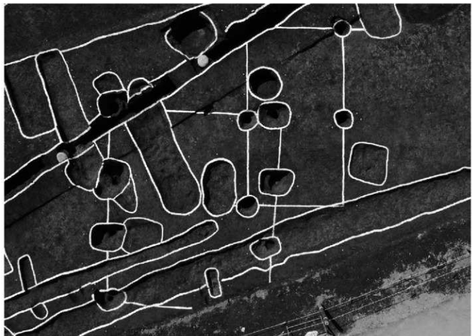
2. 3区1・3号掘立柱建物全景(上空から)
