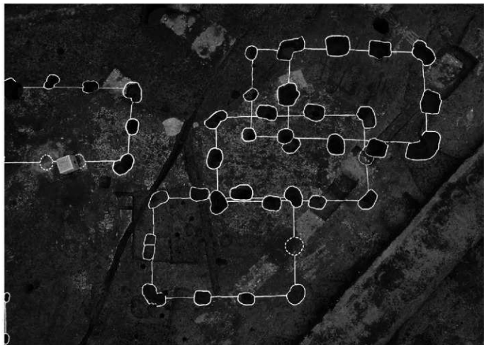
2. 1区3・5・6号掘立柱建物全景(上空から)
