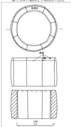
5 井戸枠実測図
