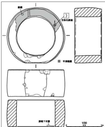
2 井戸枠実測図
