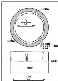
4 井戸側実測図
