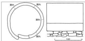
9 井戸枠・側略測図
