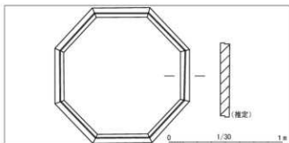
1 井戸側実測図
