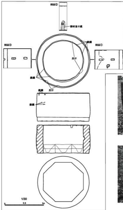
2 井戸枠実測図
