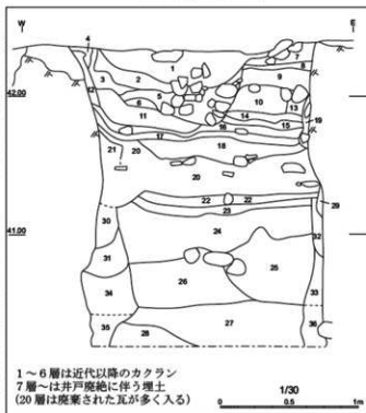
6 河北門 SE001 断面図
