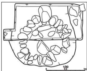
3 井戸跡 (石組) 実測図 (三ノ丸第2次 SE01)
