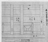
図-3 「造作弁図解」 「真之二重塀下地内之方」ほか
