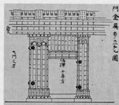
図-14.2 「来因略記」の図
