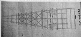
図-6 「造作弁図解」同塀橋木組立上ヨリ見ル図
