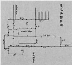
図-12 「来因略記」辰巳御櫓指図
