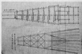
図-7 「愛本橋建築之図」より
