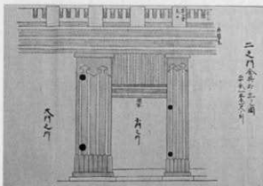
図-14.1 「造作弁図解」の図
