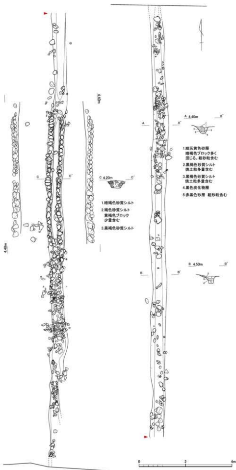
第204図 SD142(1/80)
