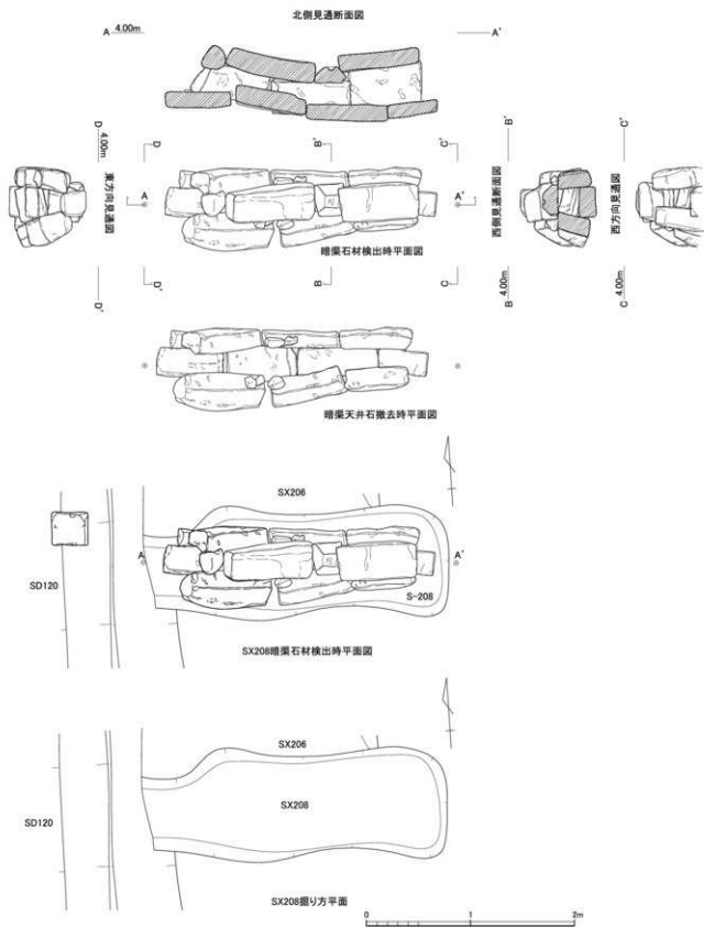
第258図 SX208 (1/40)
