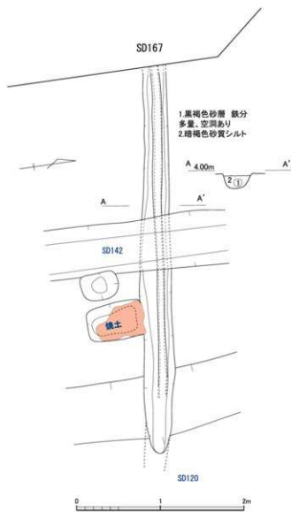
第214図 SD167 (1/40)
