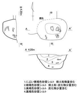
第234図 SK015(1/40)
