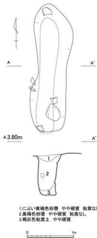
第222図 SD193(1/40)
