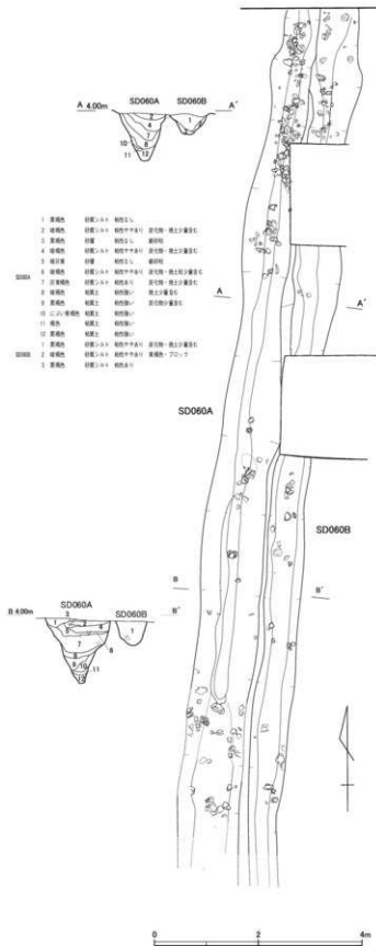
第272図 SD060A SD060B(1/80)
