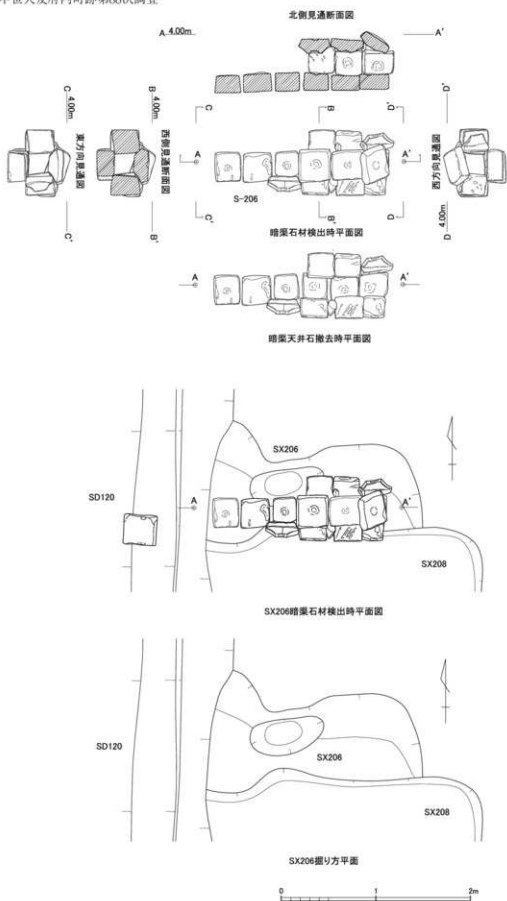
第257図 SX206(1/40)
