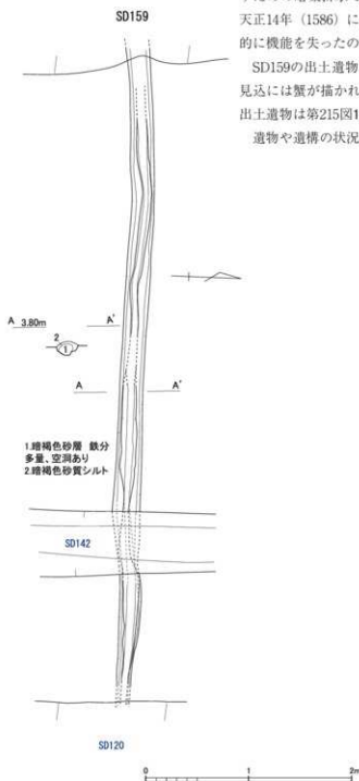
第212図 SD159(1/40)
