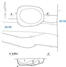
第241図 SK220(1/40)
