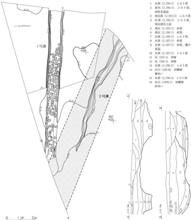
第15図 1区1・2号溝
