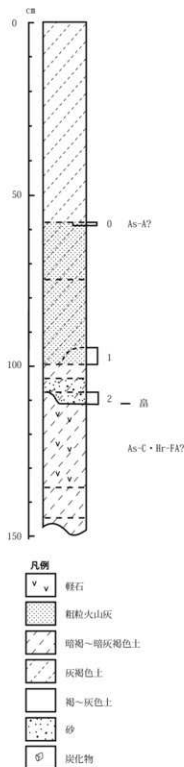
第 32 図 新島遺跡 1 区の土層柱状図 (数字はテフラ分析の試料番号)
