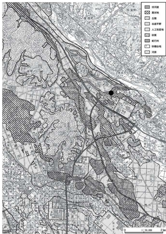
第9図 道神周辺地形分類図（群馬県「土地分類基本調査」深谷（1991）桐生及足利（1997）による）
