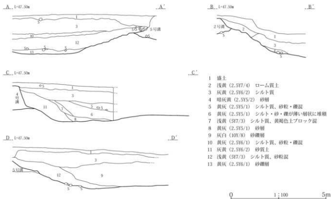
第17図 1区3号溝断面図
