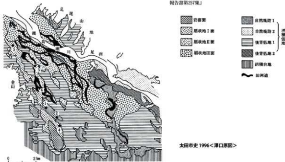
第8図 渡良瀬川扇状地の地形分類図
