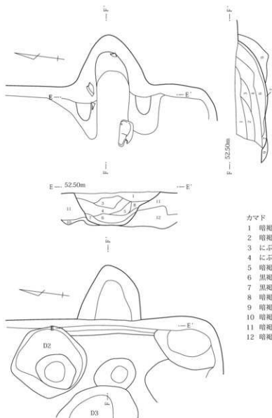
第76図 169号住居カマド
