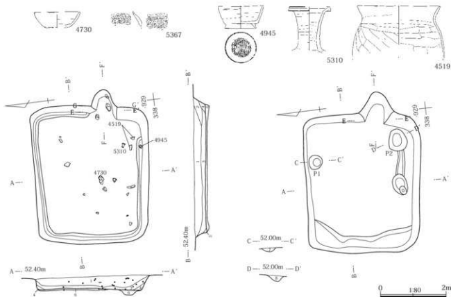
第218図 492号住居出土遺物・使用面・掘り方
