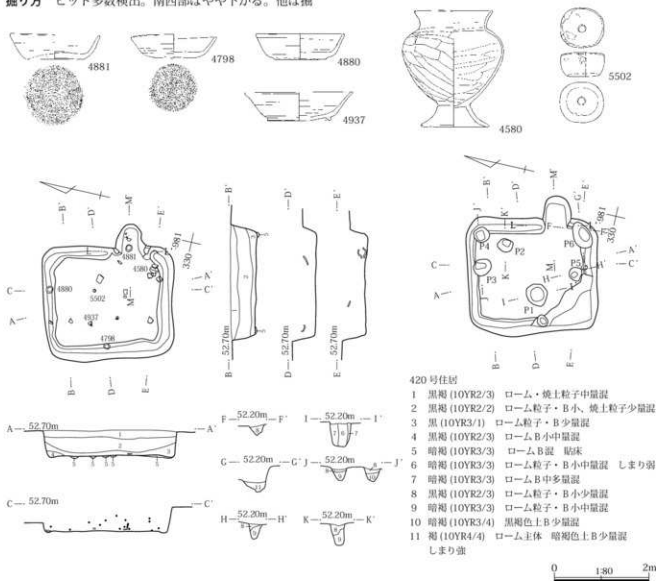
第147図 420号住居出土遺物・使用面・掘り方
