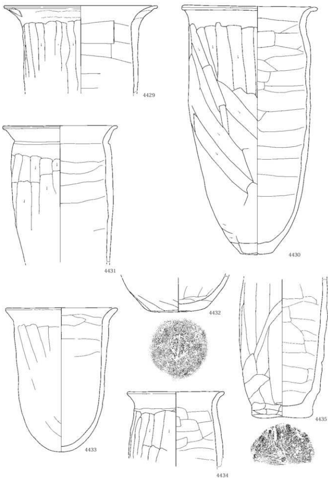
第 366 図 古墳時代後期～平安時代出土遺物 28
