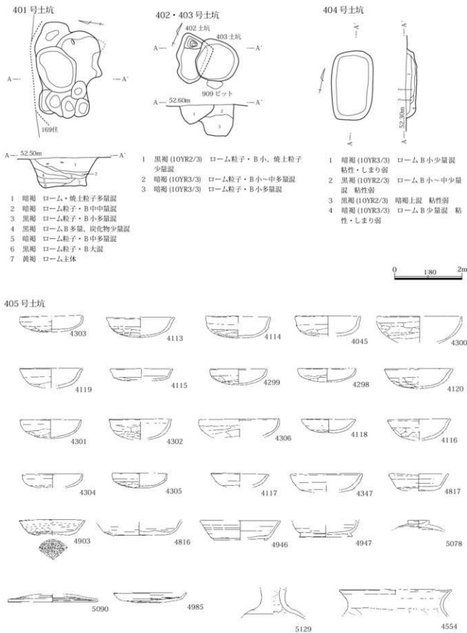
第283図 401～404号土坑 405号土坑出土遺物
