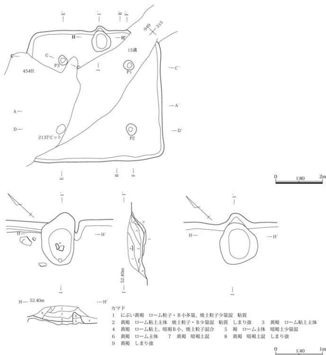
第200図 455号住居掘り方・カマド
