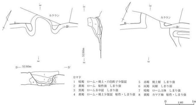
第136図 413号住居カマド
