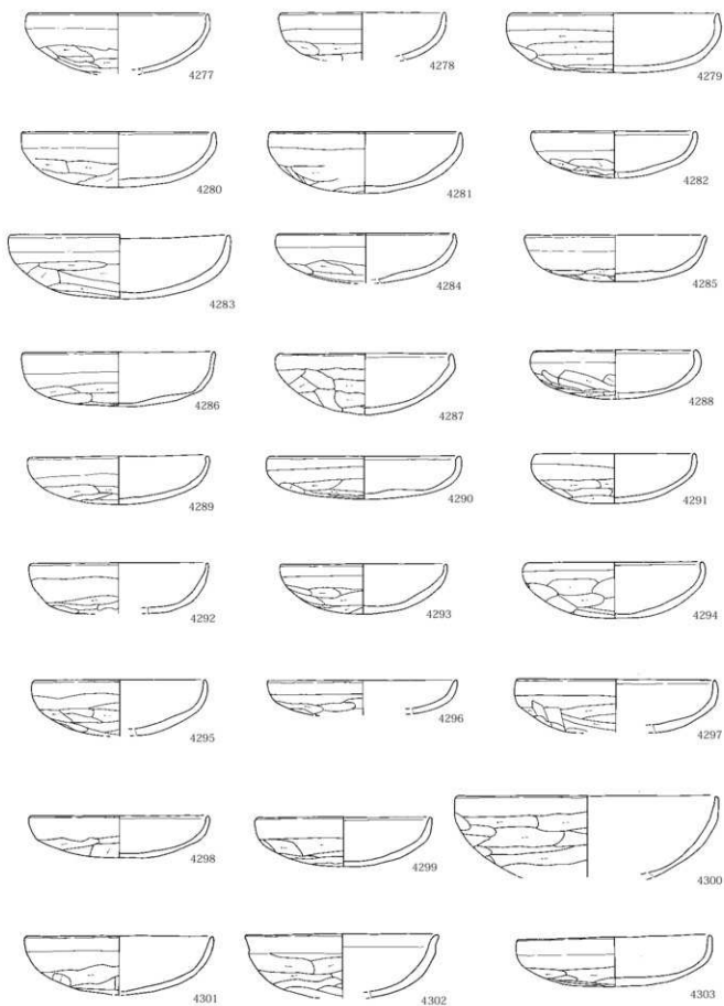
第 350 図 古墳時代後期～平安時代出土遺物 12
