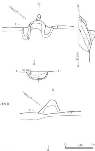
第45図 151号住居掘り方・カマド
