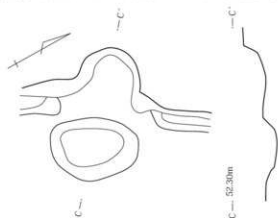
第208図 470号住居カマド
