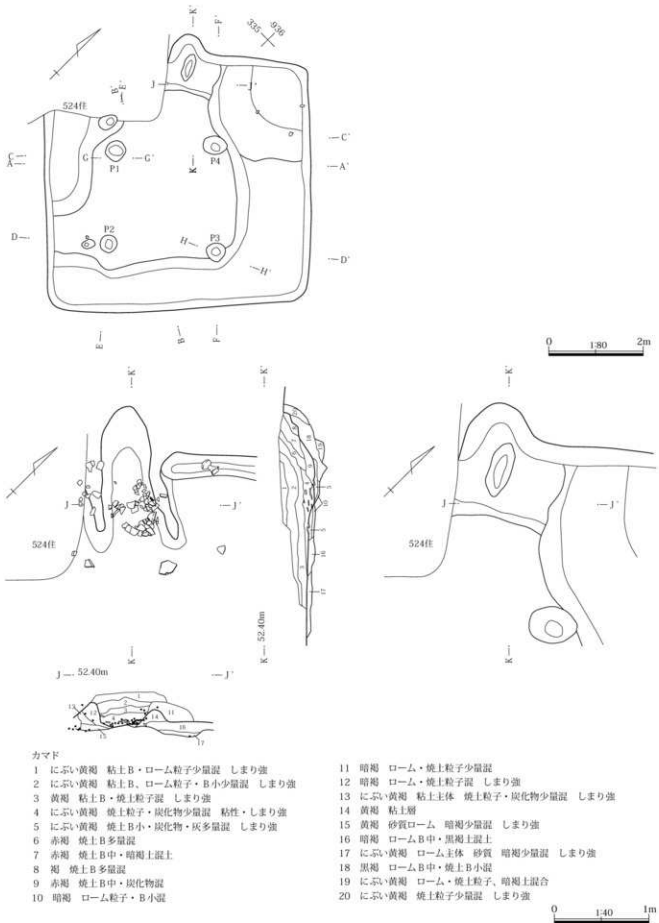
第247図 522号住居掘り方・カマド
