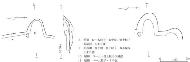
第138図 414号住居新カマド
