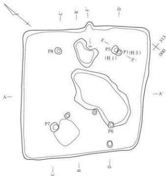
第150図 421号住居使用面・掘り方・カマド
