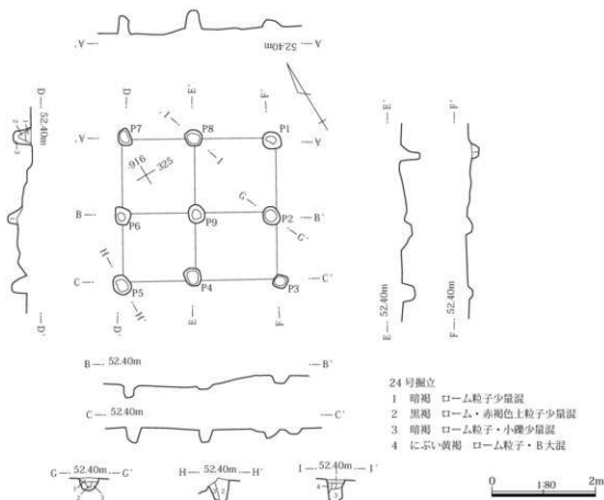
第276図 24号掘立柱建物
