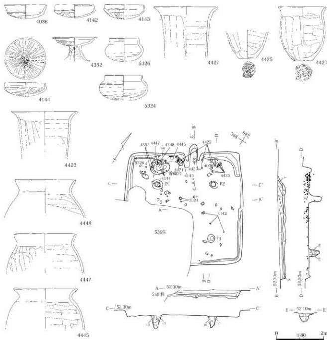
第267図 544号住居出土遺物・使用面
