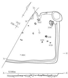
第81図 174号住居出土遺物・使用面
