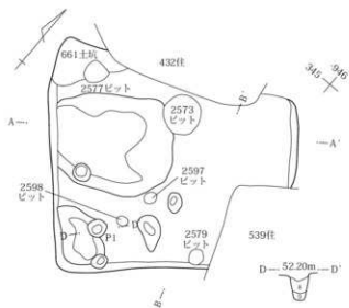
第265図 541号住居掘り方
