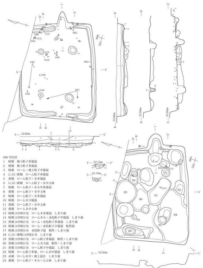
第70図 166号住居使用面・掘り方
