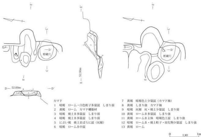
第53図 157号住居カマド
