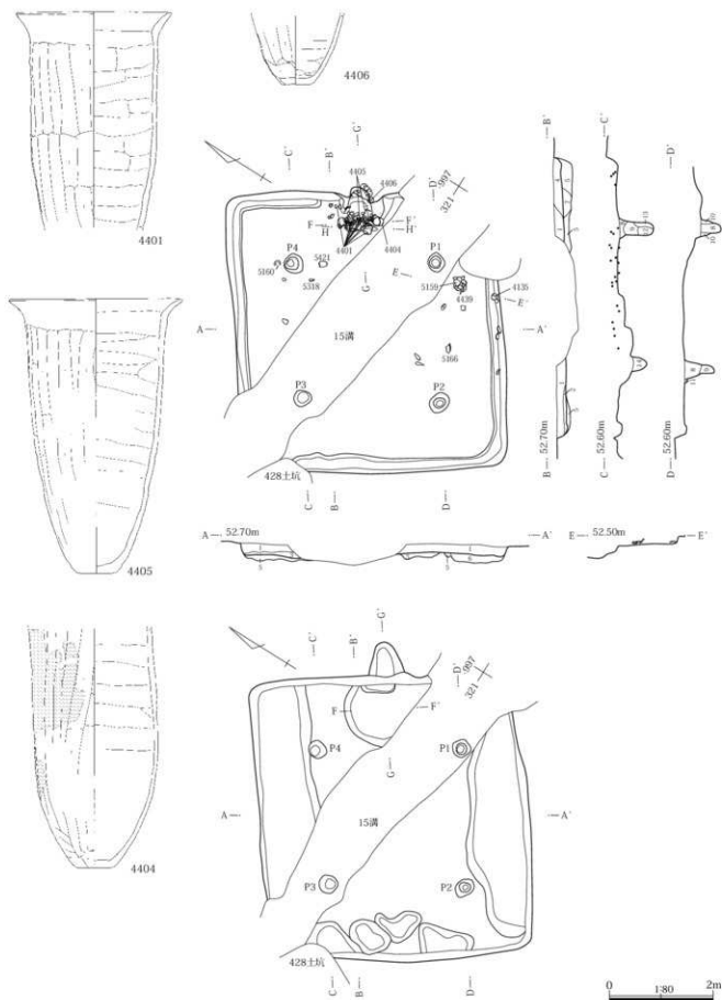
第171図 434号住居出土遺物(2)・使用面・掘り方
