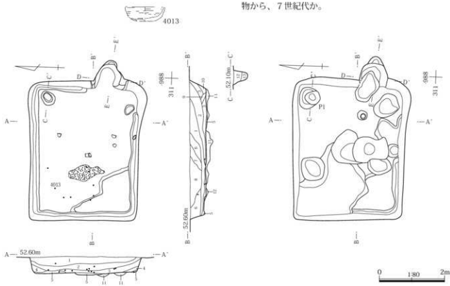
第153図 423号住居出土遺物・使用面・掘り方
