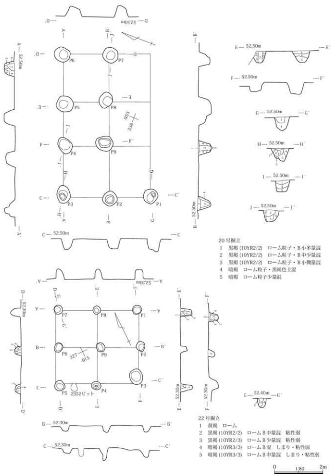
第275図 20・22号掘立柱建物
