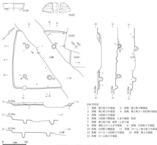
第259図 536号住居出土遺物・使用面
