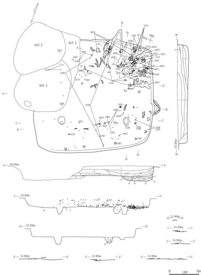
第41図 149号住居使用面
