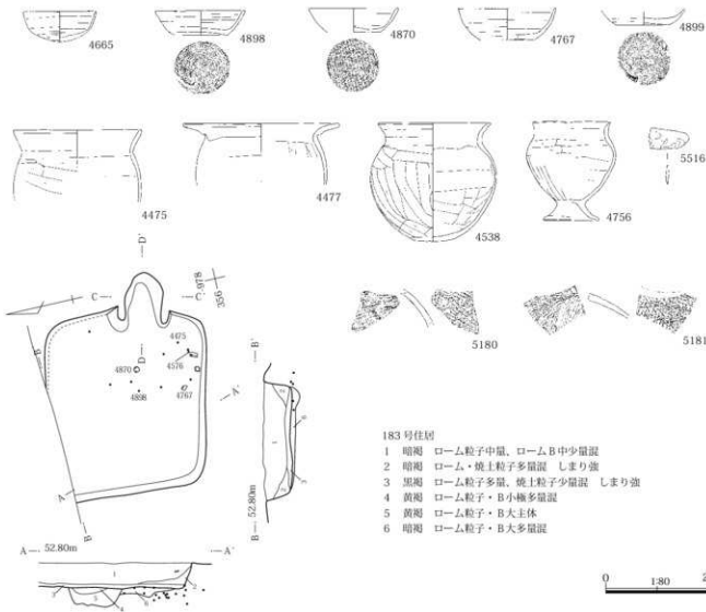
第95図 183号住居出土遺物・使用面
