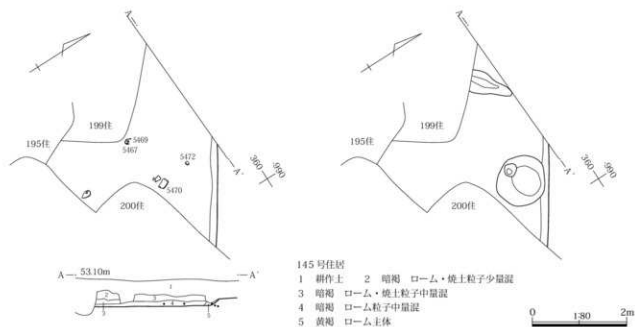
第36図 145号住居使用面・掘り方
