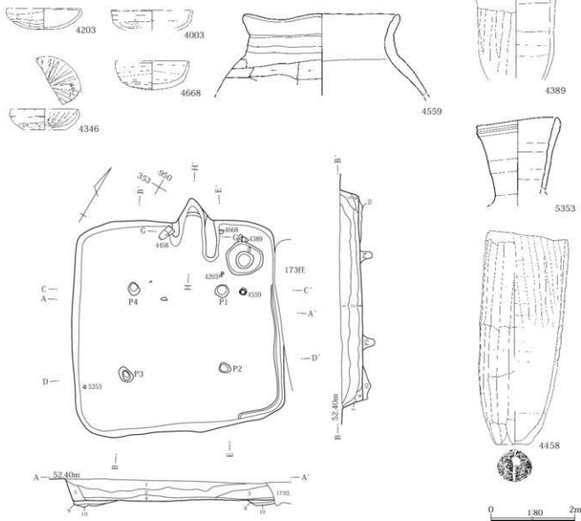
第63図 162号住居出土遺物・使用面
