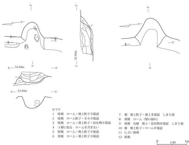
第219図 492号住居カマド
