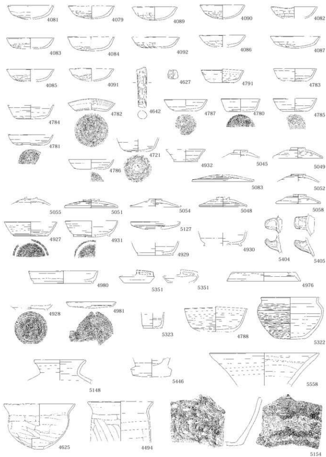
第39図 149号住居出土遺物(2)
