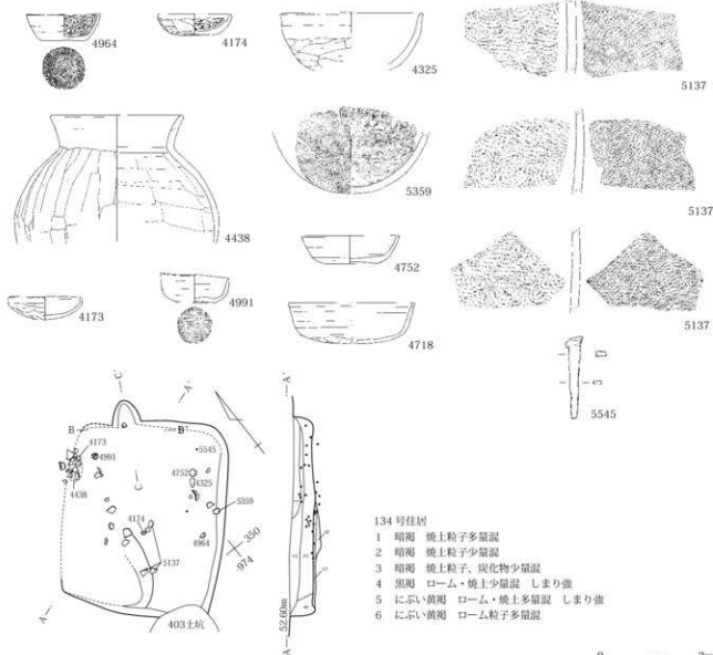
第24図 134号住居出土遺物・使用面
