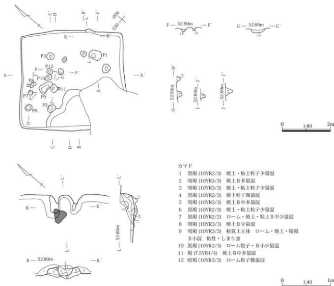
第167図 431号住居掘り方・カマド
