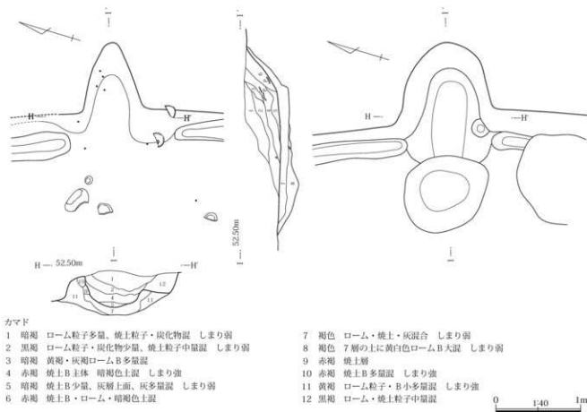
第71図 166号住居カマド
