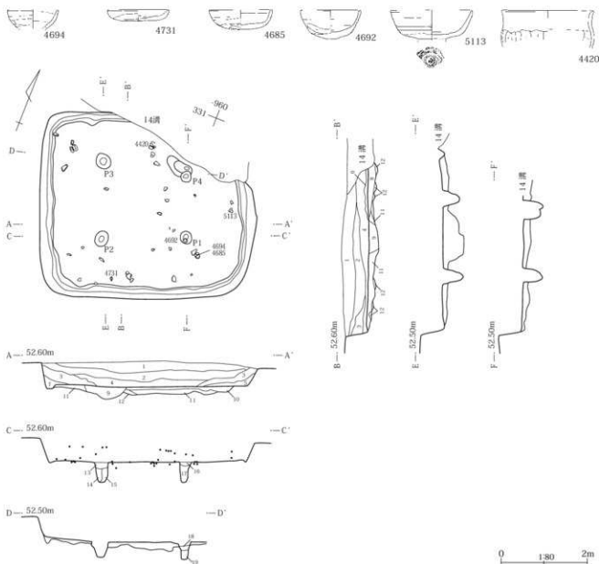
第243図 520号住居出土遺物・使用面
