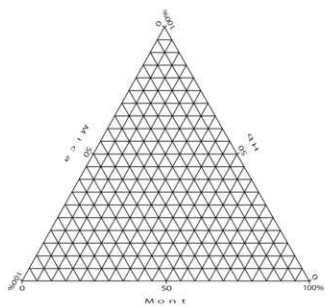
第3図 Mo-Mi-Hb 三角ダイヤグラム
