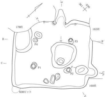
第98図 184号住居使用面・掘り方
