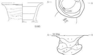
第289図 455～457・459～461号土坑 455・456・460・461号土坑出土遺物
