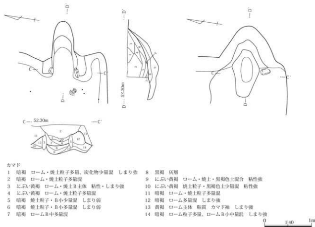
第89図 178号住居カマド
