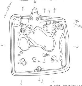
第163図 429号住居出土遺物・使用面・掘り方
