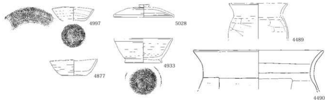
第114図 195住居出土遺物
