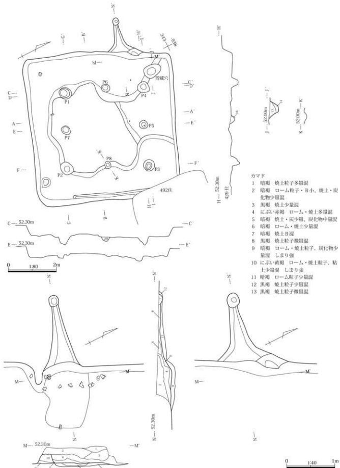
第242図 519号住居掘り方・カマド
