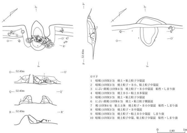
第231図 498号住居カマド
