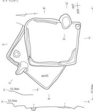
第203図 463・464号住居
