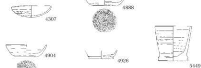
第286図 429・432・433号土坑 433・434号土坑出土遺物
