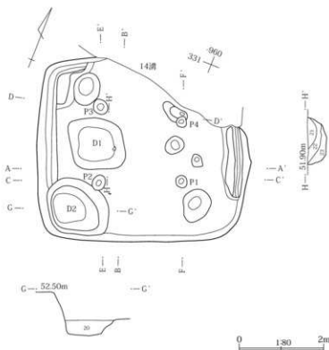
第244図 520号住居掘り方
