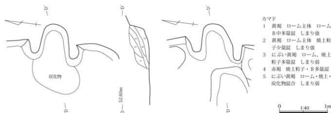
第121図 200号住居カマド
