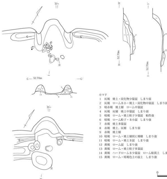
第14図 124号住居カマド
