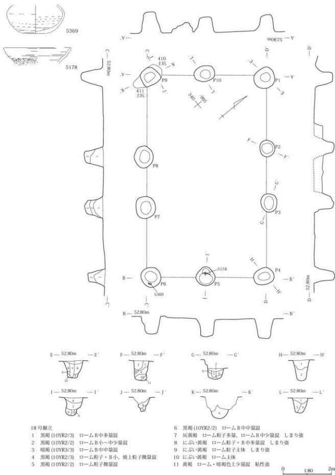
第273図 18号掘立柱建物
