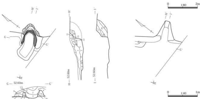
第152図 422号住居使用面・掘り方・カメラ
