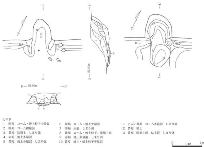
第261図 539号住居カマド
