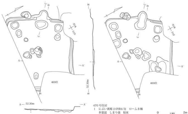
第207図 470号住居使用面・掘り方
