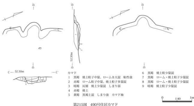
第215図 490号住居カマド
