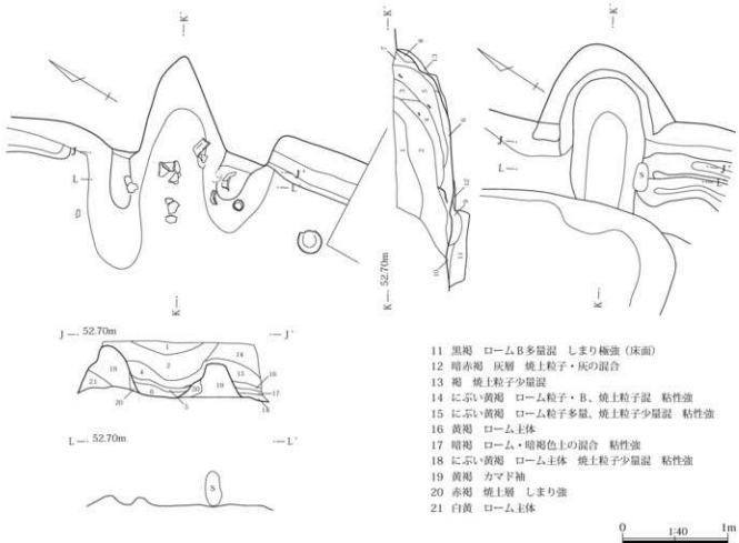
第 102図 185号住居掘り方・カマド
