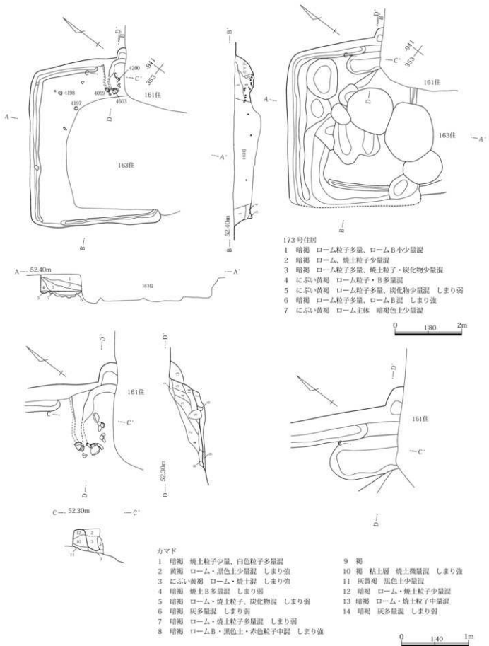
第80図 173号住居使用面・掘り方・カマド
