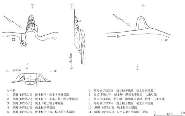
第160図 427号住居カマド
