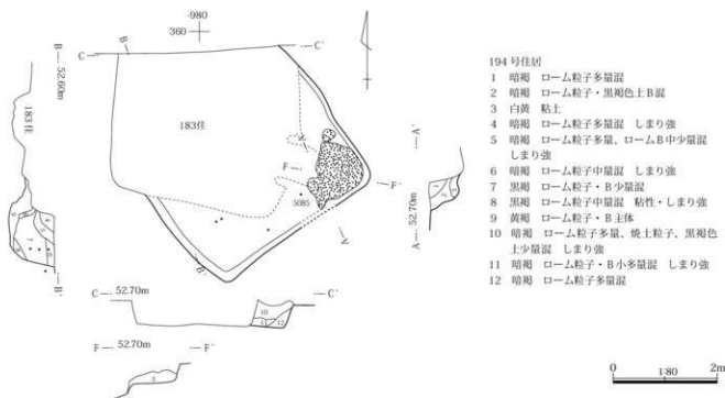
第113図 194号住居使用面
