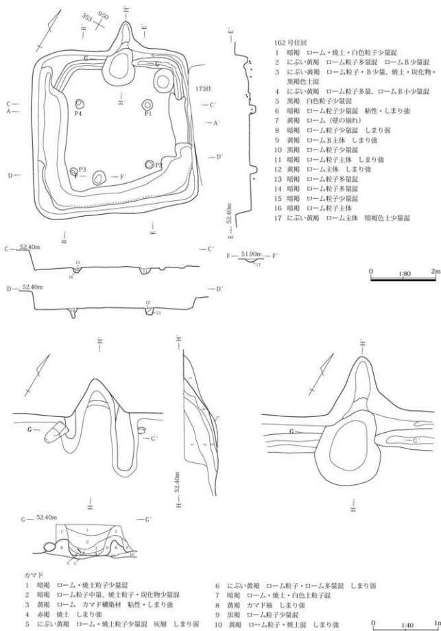
第64図 162号住居掘り方・カマド
