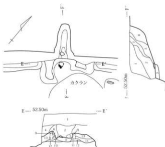
第157図 425号住居カマド
