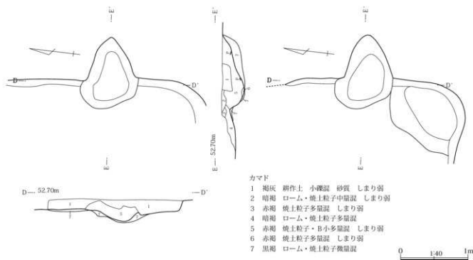
第84図 175号住居カマド
