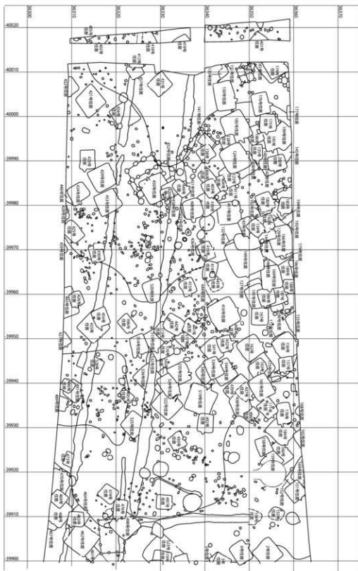
第9図 1・2区整穴住居配置図
