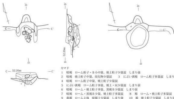
第213図 489号住居カマド
