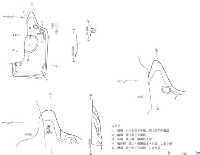
第27図 135号住居掘り方・カマド
