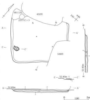
第264図 541号住居使用面
