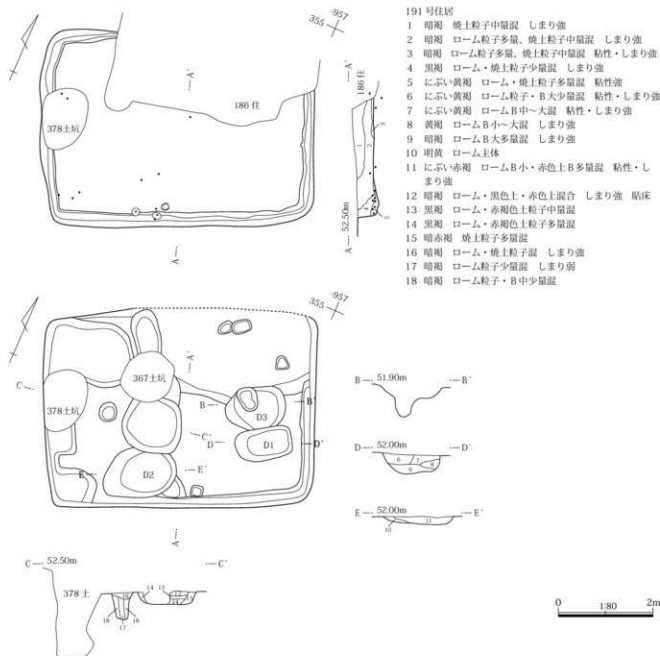
第110図 191号住居使用面・掘り方
