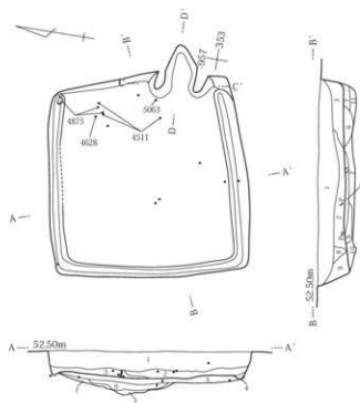
第103図 186号住居出土遺物・使用面・掘り方
