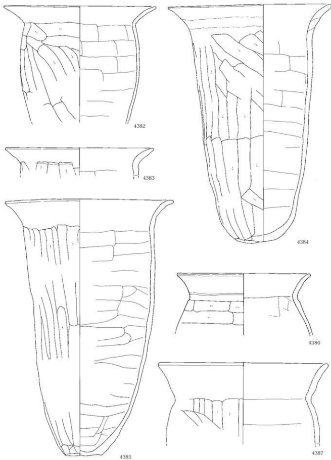
第 358 図 古墳時代後期～平安時代出土遺物 20
