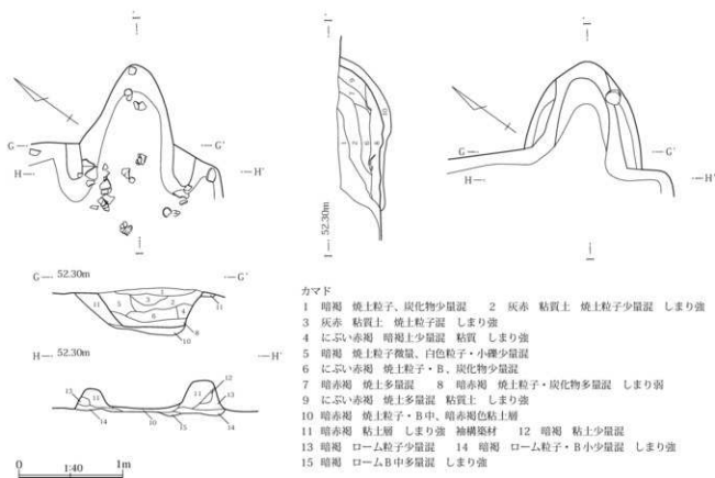
第237図 515号住居カマド
