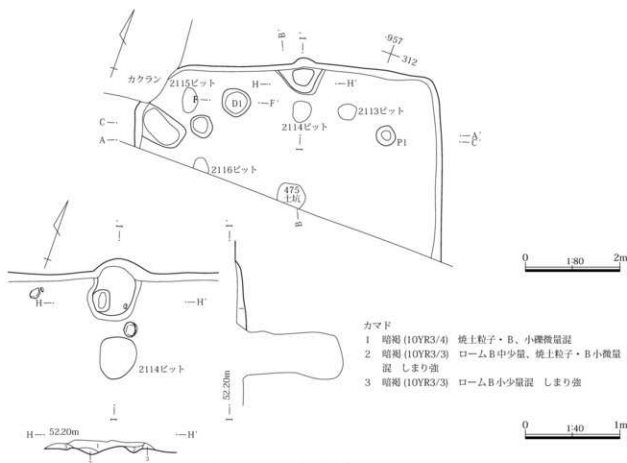
第186図 443号住居掘り方・カマド
