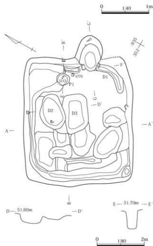
第62図 161号住居掘り方・カマド
