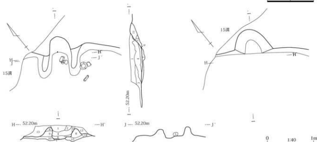
第217図 491号住居使用面・掘り方・カマド
