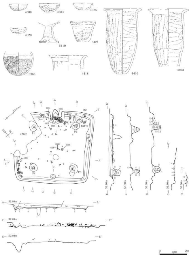
第229図 498号住居出土遺物・使用面
