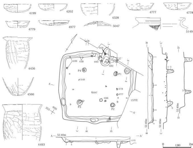
第50図 156号住居出土遺物・使用面
