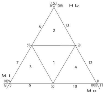
第1図 三角ダイヤグラム、位置分類図
