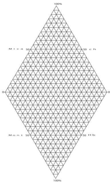
第4図 Mo-Mi-Hb-CH 菱角ダイヤグラム
