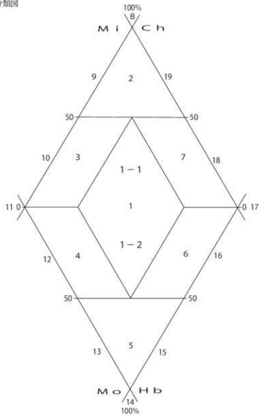
第2図 菱形ダイヤグラム、位置分類図
