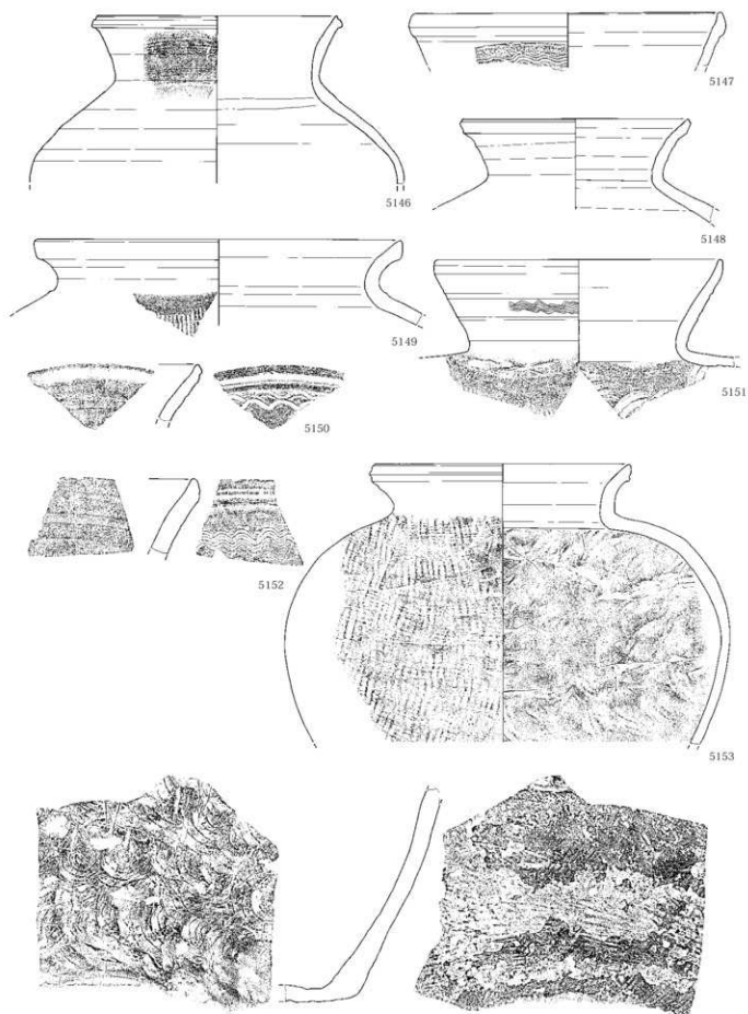
第 419 圖 古墳時代後期～平安時代出土遺物 81
