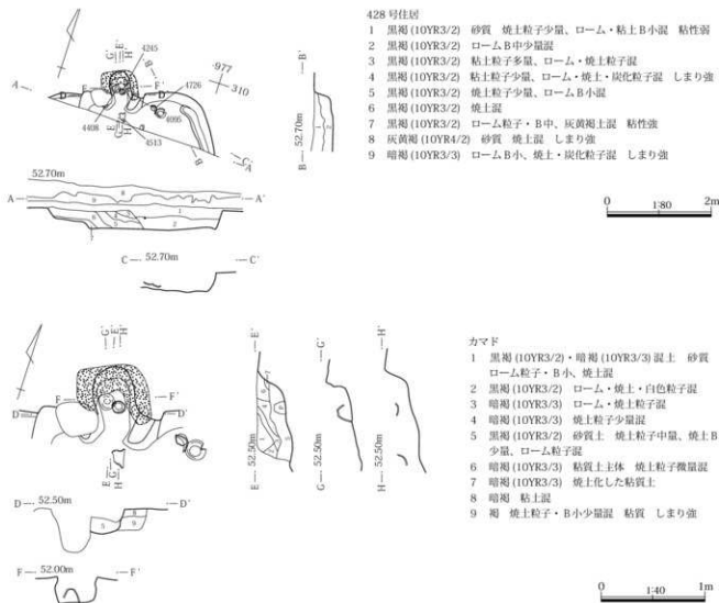
第162図 428号住居使用面・カマド
