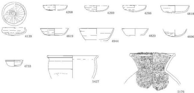
第248図 524号住居出土遺物(1)
