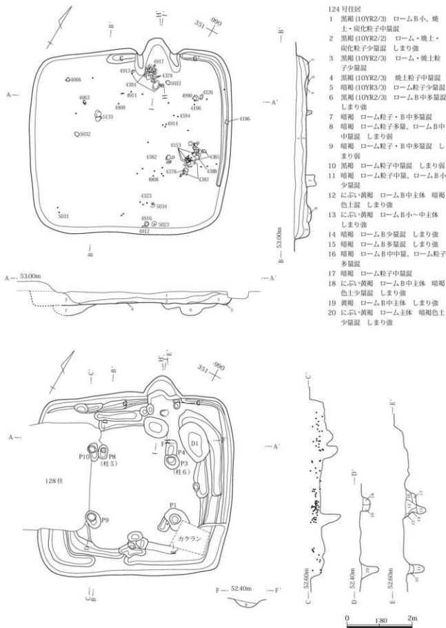
第13図 124号住居使用面・掘り方
