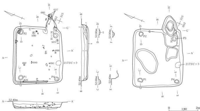
第197図 454号住居出土遺物・使用面・掘り方
