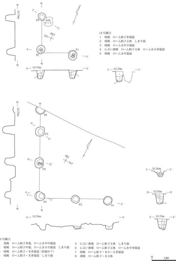
第271図 14・15号掘立柱建物
