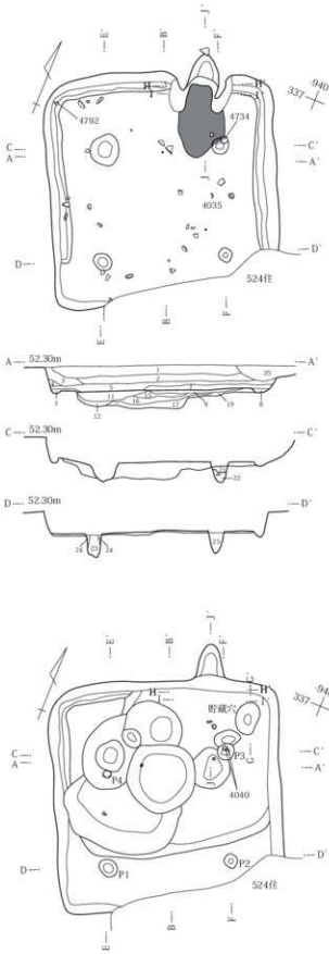
第256図 535号住居使用面・掘り方
