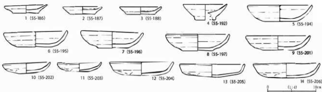
図215 55SK41詳細図
