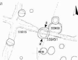
図216 55SK51平面・断面図
