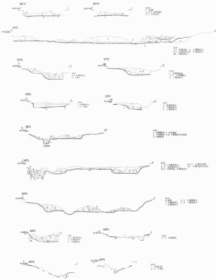
図172 23SG1断面図(2)
