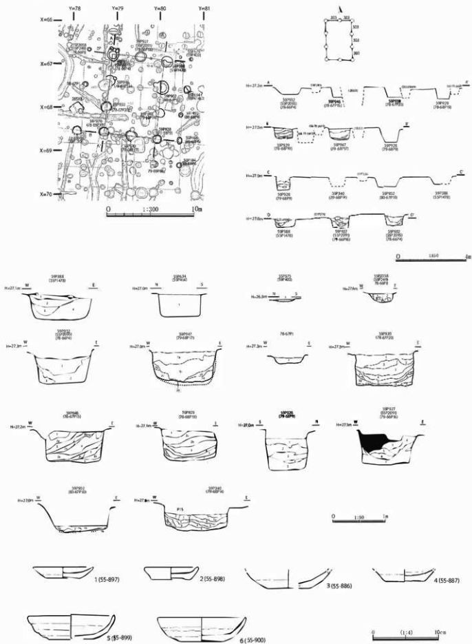
図83 28SB6詳細図
