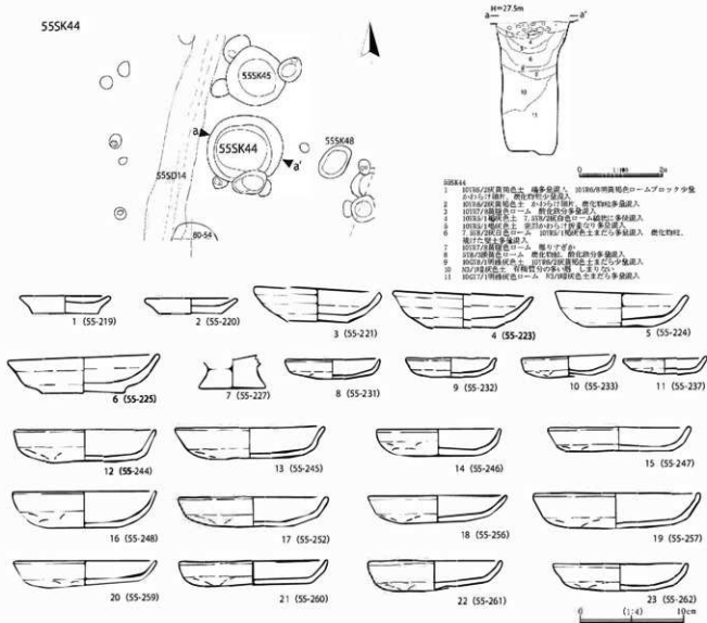
図191 55SK44詳細図
