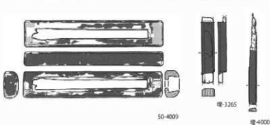
図285 木製品実測図(5)
