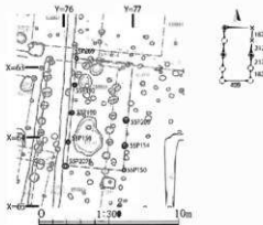
図145 55SB29平面図
