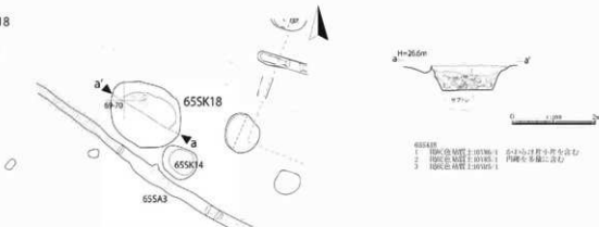
図240 65SK18平面・断面図
