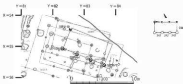
図134 55SB14平面図
