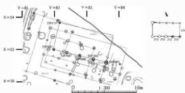
図133 55SB13平面図
