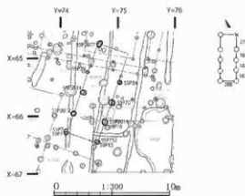
図141 55SB23平面図
