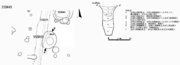
図190 55SK43平面・断面図
