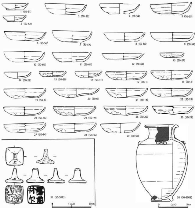
図180 50SE3詳細図
