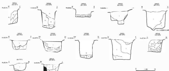
図79 28SB3詳細図
