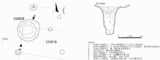
図189 55SK38平面・断面図
