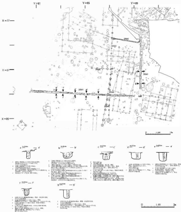
図249 23SA1平面・断面図
