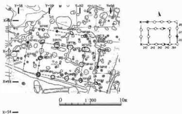
図146 56SB1平面図
