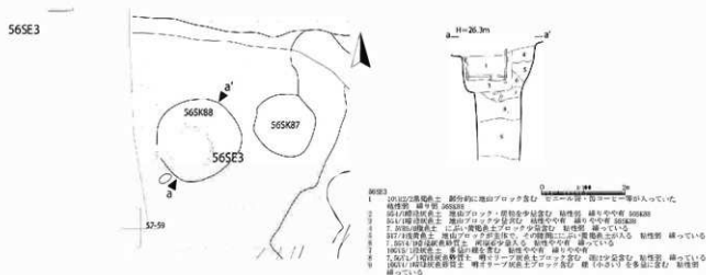
図193 56SE3平面・断面図
