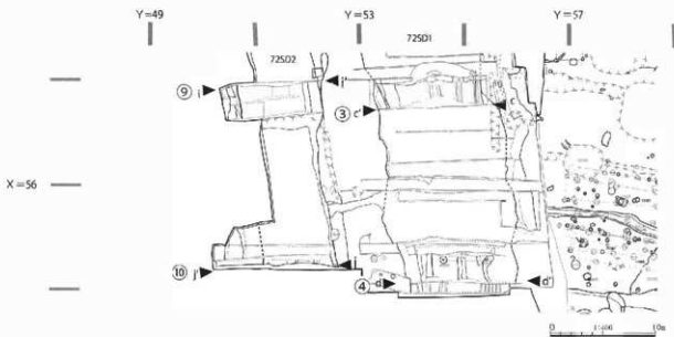
図57 遺跡北端部72SD1・72SD2平面図 (1/400)
