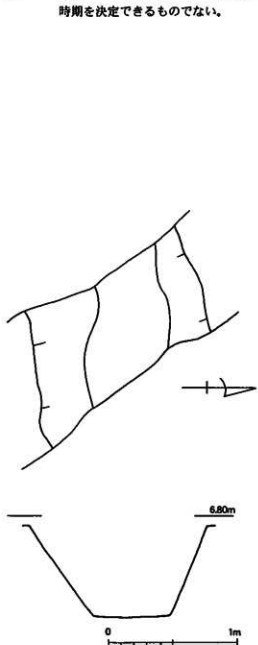
第8図 府内町跡61次調査Ⅰ区 SD114実測図
