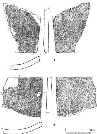
第17図 府内町跡61次調査Ⅰ区出土瓦実測図(2)
