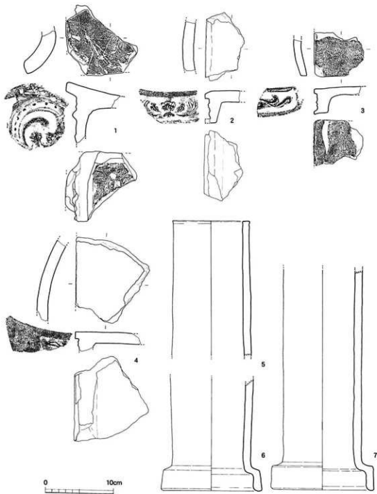
第33図 府内町跡61次調査Ⅱ区表土・表探遺物実測図(2)
