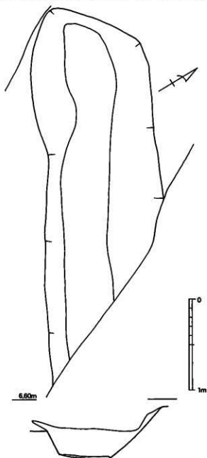
第9図 府内町跡61次調査Ⅰ区 SD115実測図
