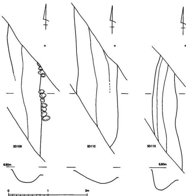
第7図 府内町跡61次調査Ⅰ区 SD109・SD112・SD113実測図
