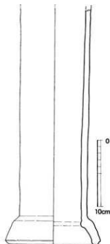
第18図 府内町跡61次調査Ⅰ区出土土管実測図
