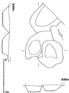
第25図 府内町跡61次調査Ⅱ区SK215実測図
