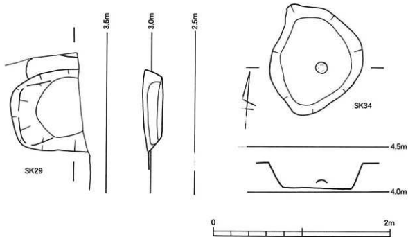
第31図 SK29・SK34実測図
