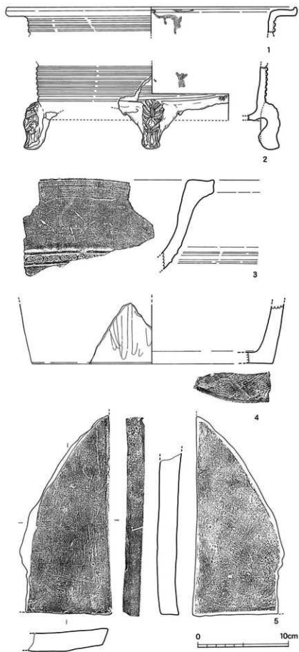
第55图 包含层出土文物实测图
