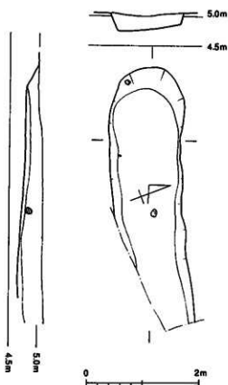
第26図 SD263実測図
