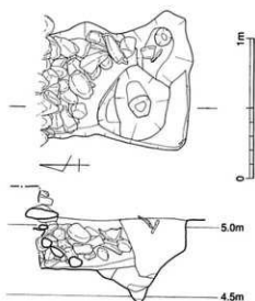
第38図 SK26実測図
