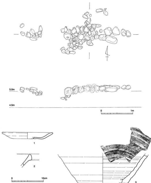
第31図 SX41遺構及び出土遺物実測図
