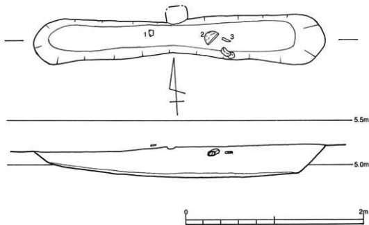
第46図 SK191実測図
