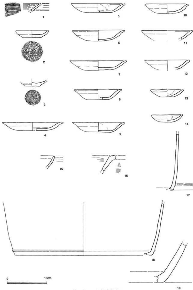
第47图 SE24 出土遺物実測図
