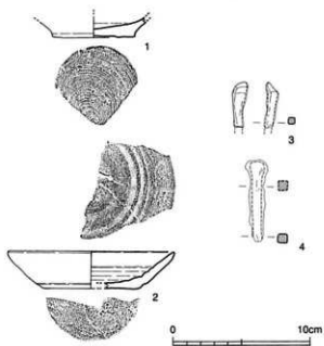
第23図 SK127出土遺物実測図
