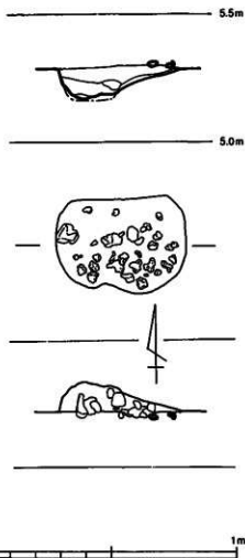
第16図 SX46実測図
