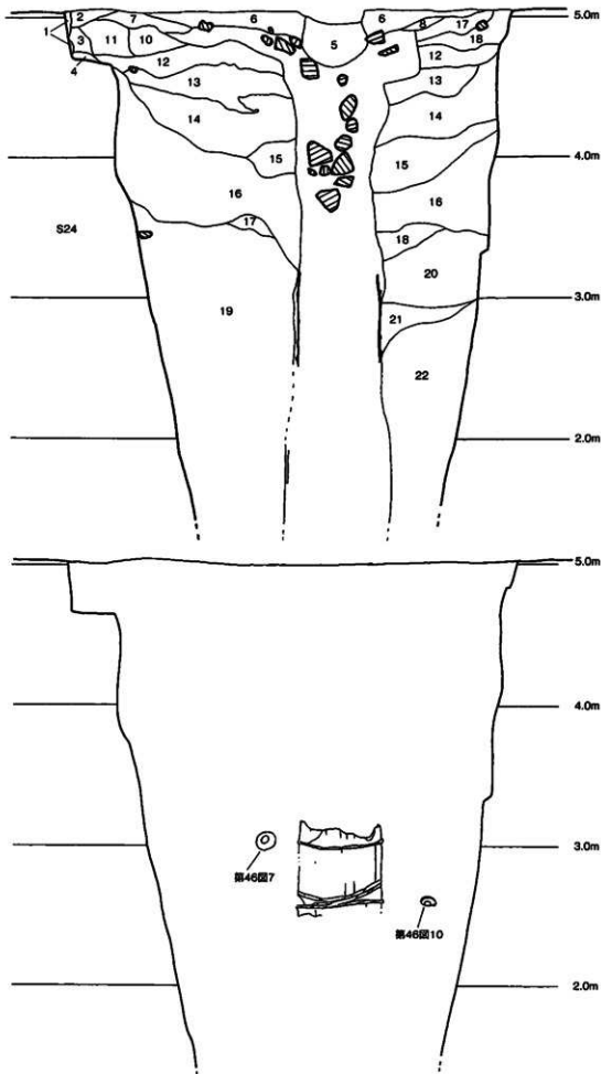
第46圖 SE24土層圖・井戸側断面圖
