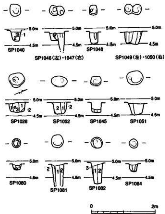
第 112 図 柱穴実測図
