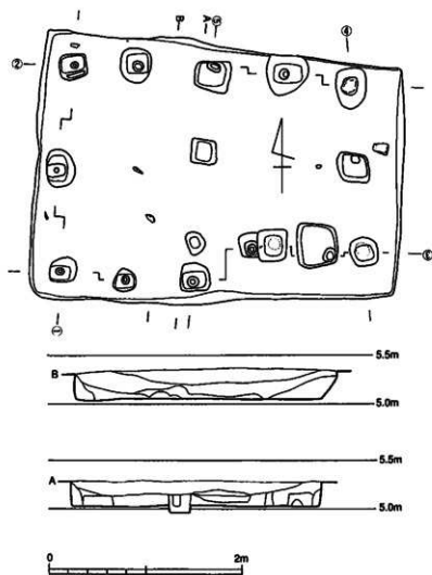
第34図 SK80土層図
