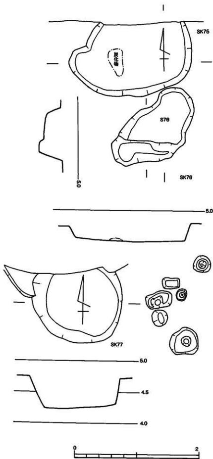
第80図 SK75～77 実測図
