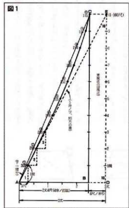
本高さ80尺(10間)4分の打出、5分ノリの割付例
