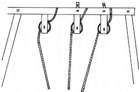
②滑車の使い方図Ⅴ
