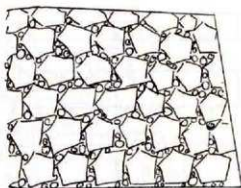
曲尺場取り残し積みの絵図
