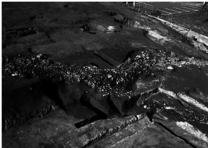
Ⅱ区1号製鉄炉 北排滓坑・排滓溝・排滓場 遺物出土状況①（南東より）
