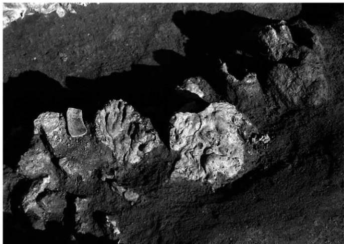
I区1号製鉄炉 第1面 遺物出土状況 (A区近景)
