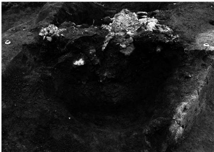
Ⅱ区1号製鉄炉 掛沖溝 土層断面A-A' (南西より)
