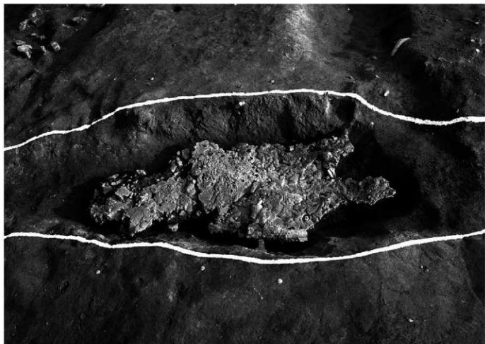
Ⅱ区2号製鉄炉 流動滓（1-288）近景（二股に別れており、小口両端の排滓孔から流れ出ていることがわかる。）
