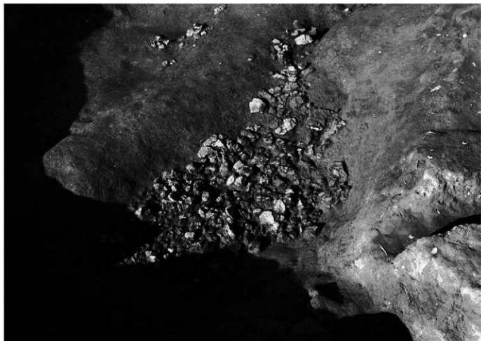
Ⅱ区2号製鉄炉 南排滓坑 遺物出土状況近接③ (東より)
