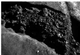
Ⅱ区1号製鉄炉 排滓溝 遺物出土状況近景③(西より)
