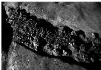
Ⅱ区1号製鉄炉 排滓溝 遺物出土状況近景①(東より)
