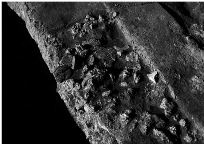
I区1号製鉄炉 第1面 遺物出土状況 (E区近景)
