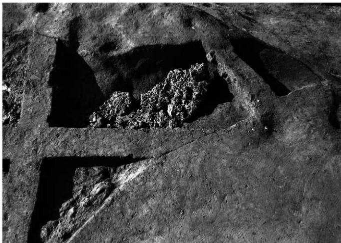
1区1号製鉄炉 第1面 遺物出土状況 (G区・H区近景)
