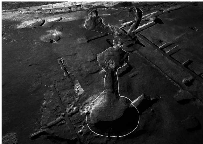
Ⅱ区1号製鉄炉 全景㉘ (南上空より)
