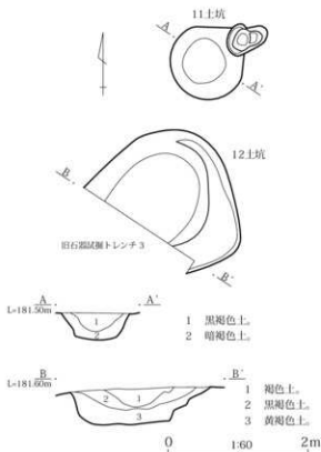
第4図 11号・12号土坑実測図
