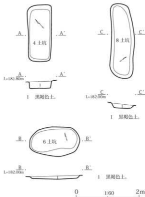
第8図 4号・6号・8号土坑実測図
