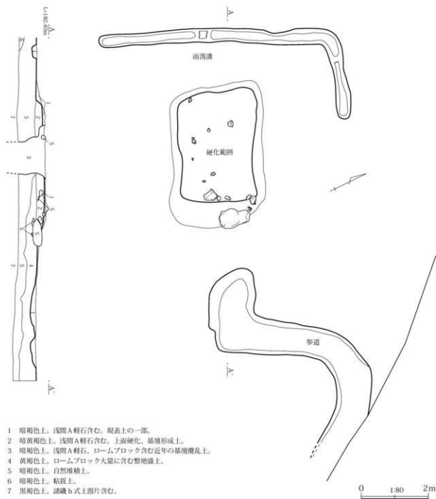
第11図 1号基壇建物実測図
