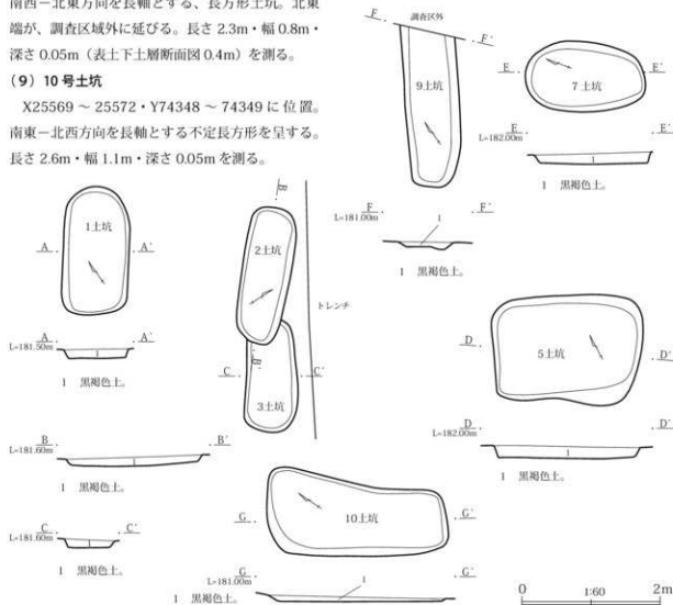
第14図 1号～3号・5号・7号・9号・10号土坑実測図
