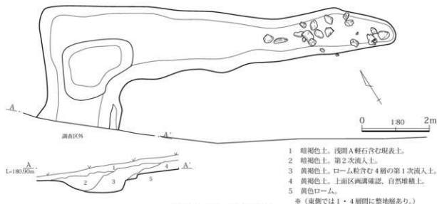
第13図 1号区画溝実測図
