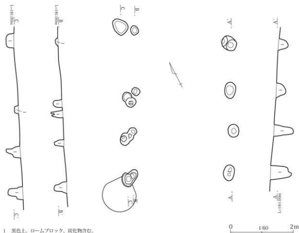
第10図 1号掘立柱建物実測図
