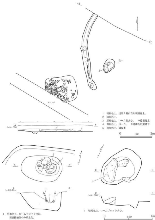
第5図 1号住居(上)・同埋竈炉(下左)・同石囲炉(下右)実測図
