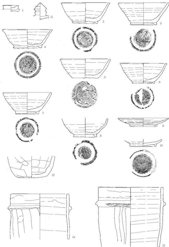
44 図 B区4号壜穴建物出土遺物図(1)
