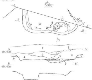
46図 B区5号竪穴建物平面図・断面図
