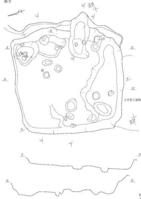
35図 B区3号竪穴建物掘方平面図・断面図
