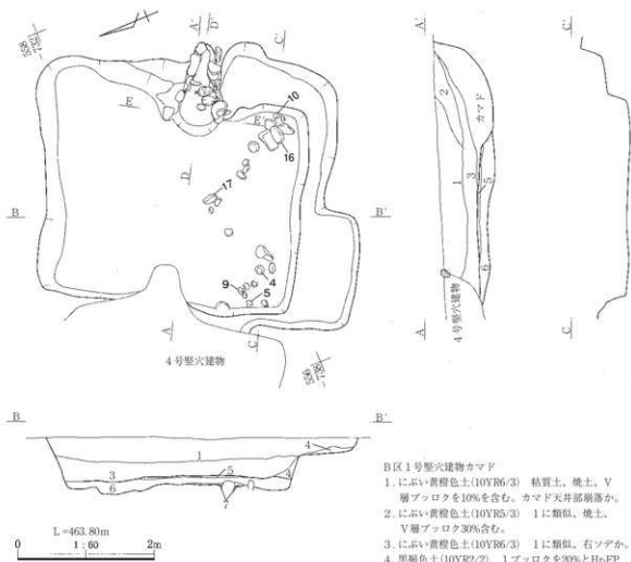
24図 B区1号型穴建物平面図・断面図
