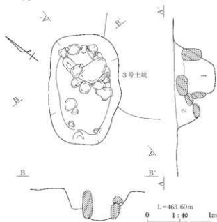
22図 B区4号土坑平面図・断面図(1)
