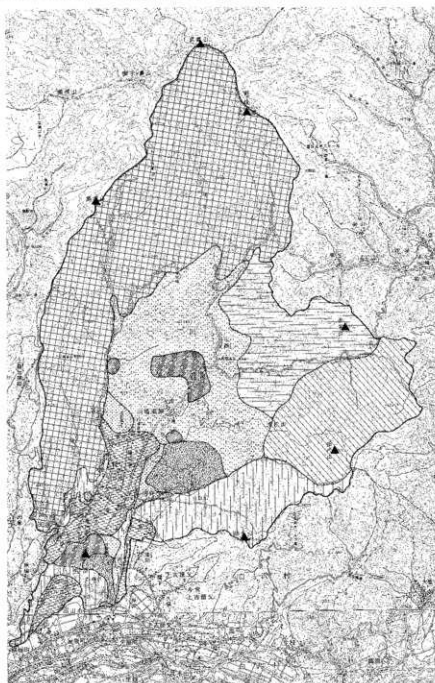
4図 川場村地質図(1/50,000)
