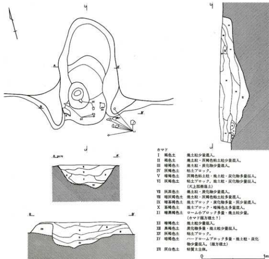
第120図 B区第45号住居跡カマド
