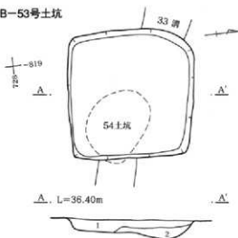
第274図 B-49号~53号土坑平・断面図
