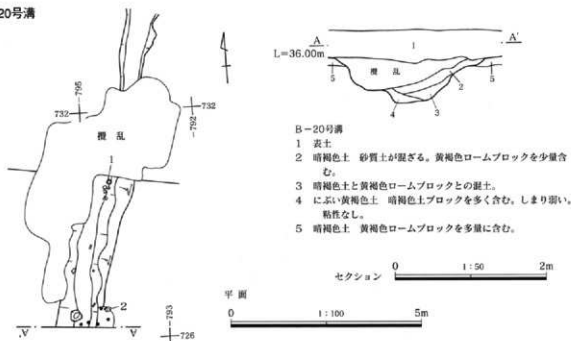
第279図 B-20号溝平・断面図
