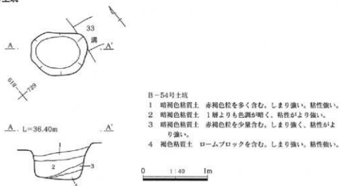
第275図 B-54号土坑平・断面図
