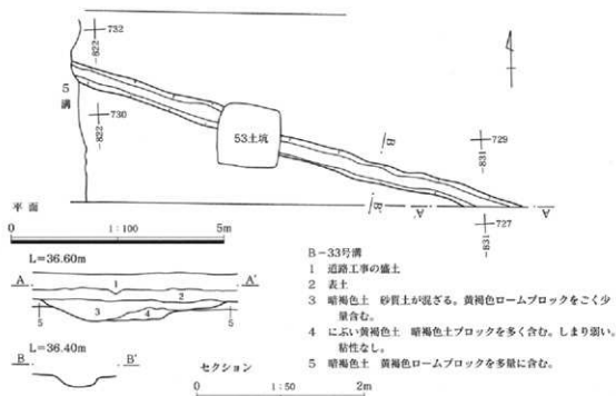
第281図 B-33号溝平・断面図
