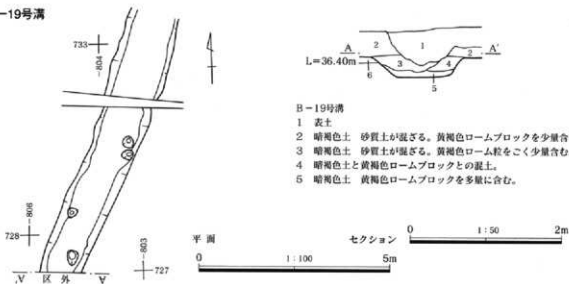
第277図 B-19号溝平・断面図
