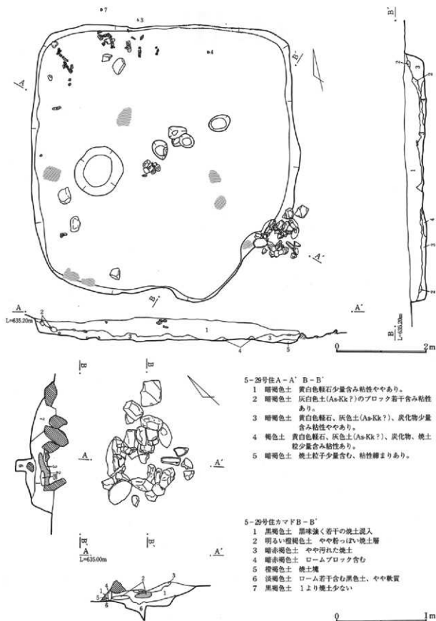
第239図 5-29号住居跡
