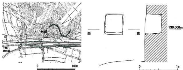
第10図 中津市耶馬溪町大島 石祠実測図
