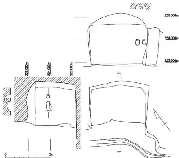
第2図 上小原地区横穴遺構実測図
