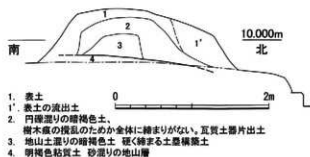
第4図 植野伽藍遺跡土塁実測図
