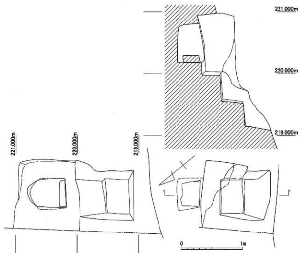
第3図 上小原地区祠遺構実測図
