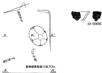
第122図 第14号住居跡 1:60・出土遺物実測図 1:3
