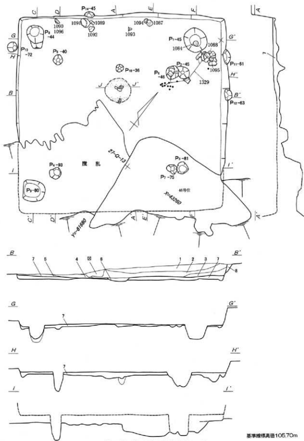
第217图 第50号住居跡実測图 1 : 60
