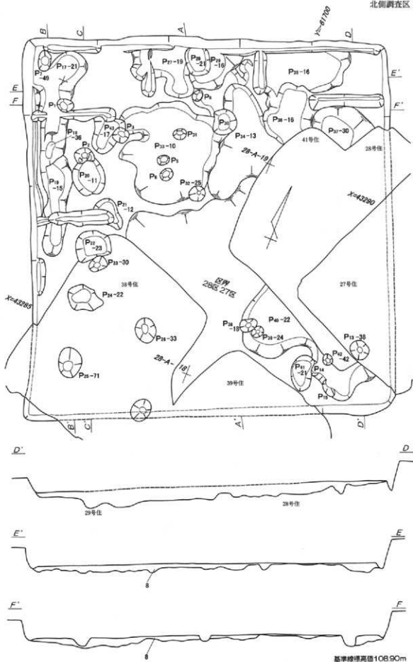
第192图 第42号住居跡掘方实测图 1 : 60
