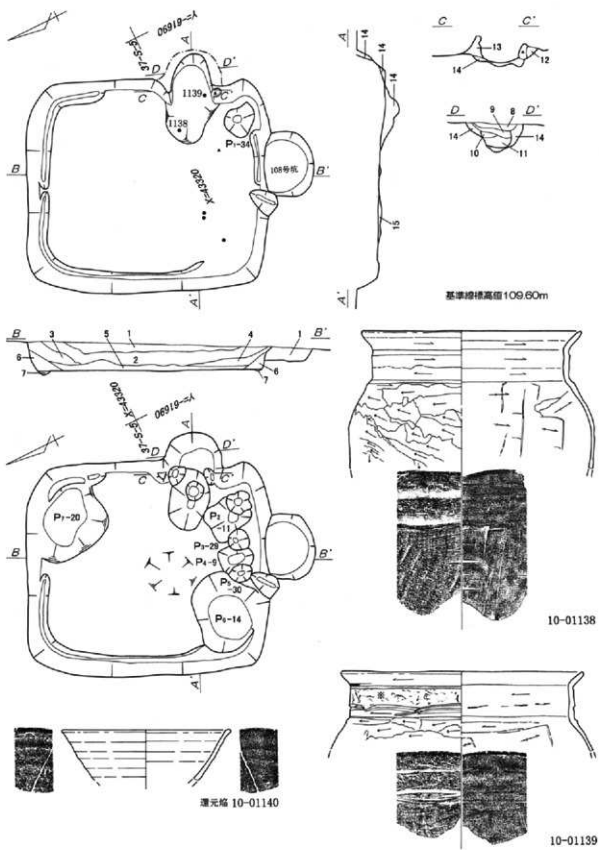
第229图 第57号住居跡 1:60・出土遺物実測図 1:3 (1)
