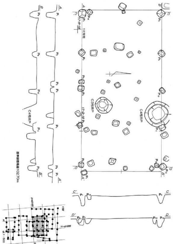
第41图 第3号掘立柱建物跡実測図 1:60
