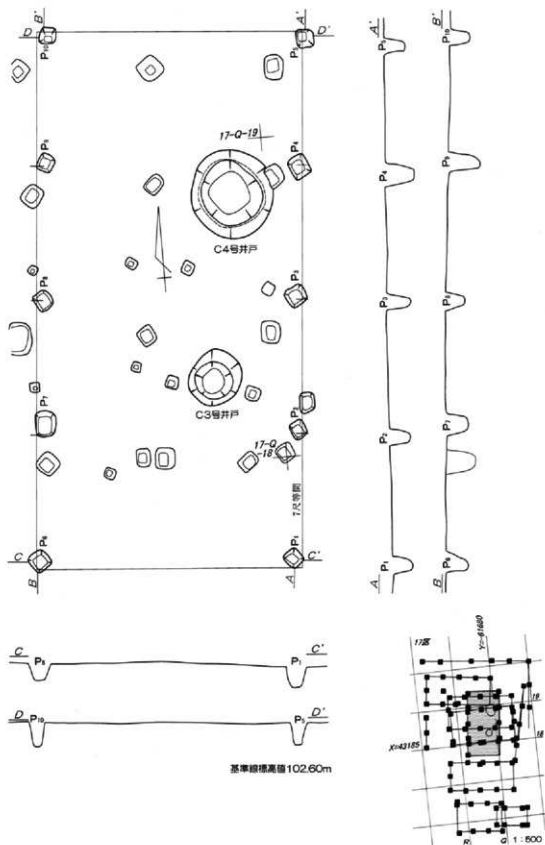
第43図 第5号独立柱建物跡実測図 1:60
