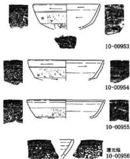
第187图 第40・59号住居跡 1 : 60・第40号住居跡出土遺物実測図 1 : 3 (1)
