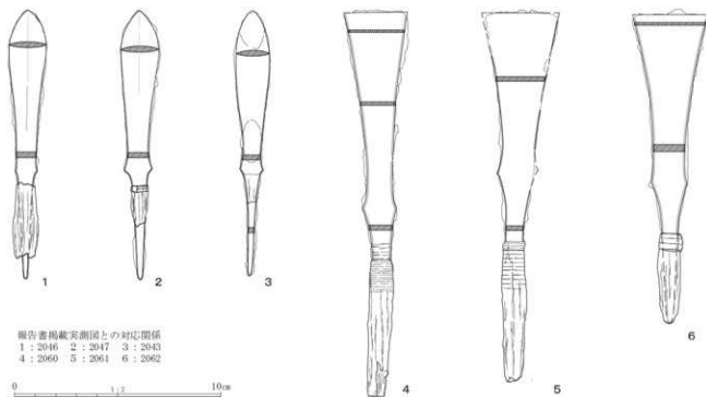
図3 小迫2号墓出土鉄器実測図
