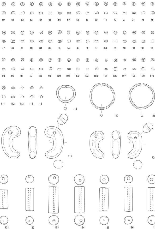
第6圖 志手金毘羅山古墳出土遺物実測圖③ (1/1)
