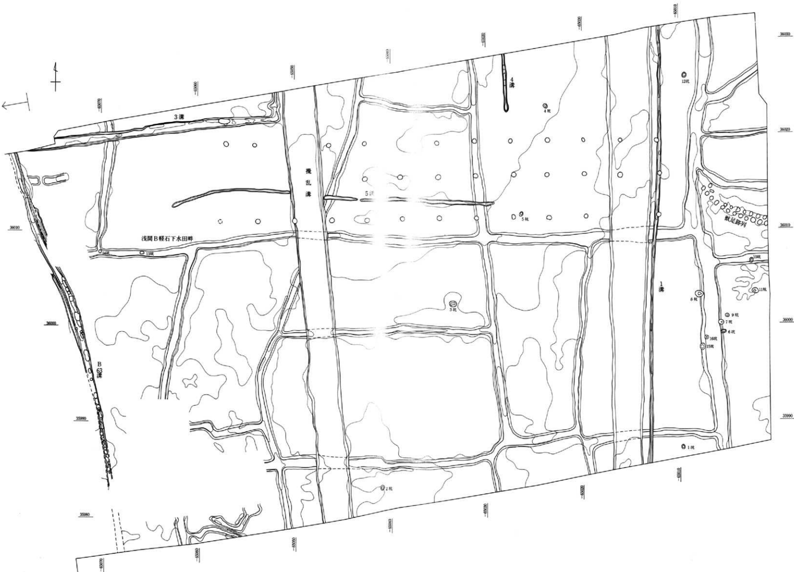
付図-3 C区遺構配置図 (1/200)
