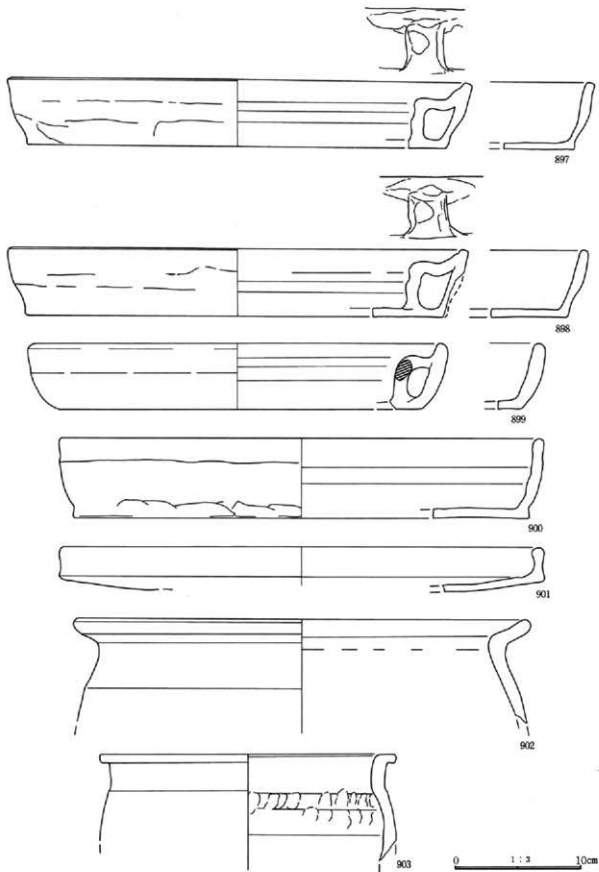
第180图 B区24号溝出土遺物 (6)
