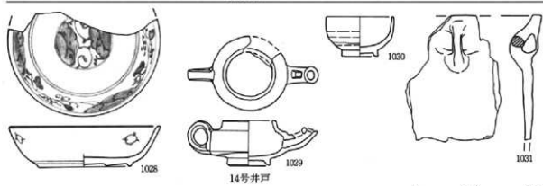
第194図 B区13・14号井戸出土遺物
