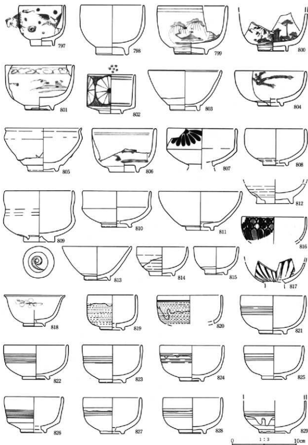
第176图 B区24号溝出土遺物(2)
