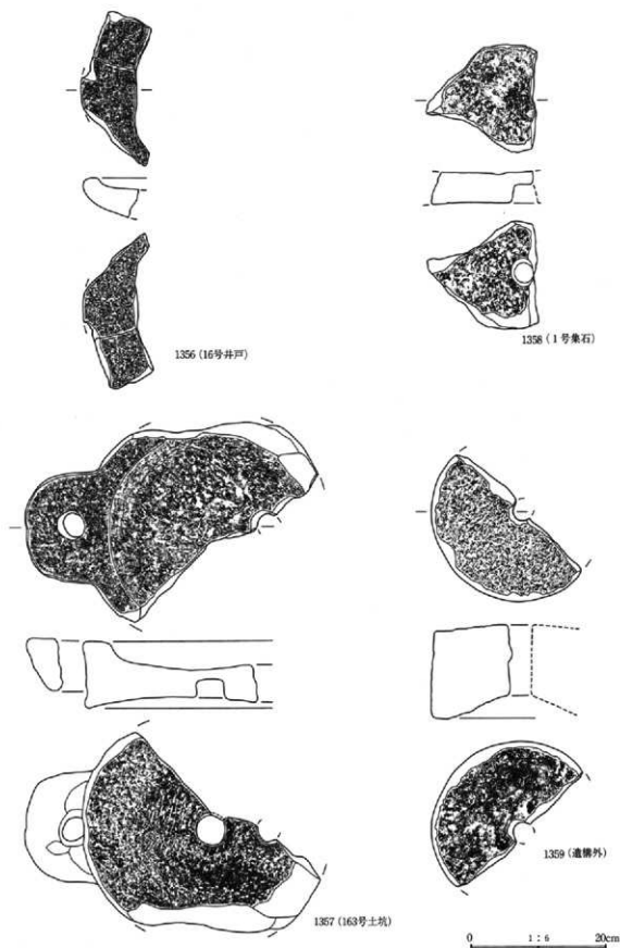
第243图 A区16号井戸、1号集石、163号土坑、遺構外出土石臼
