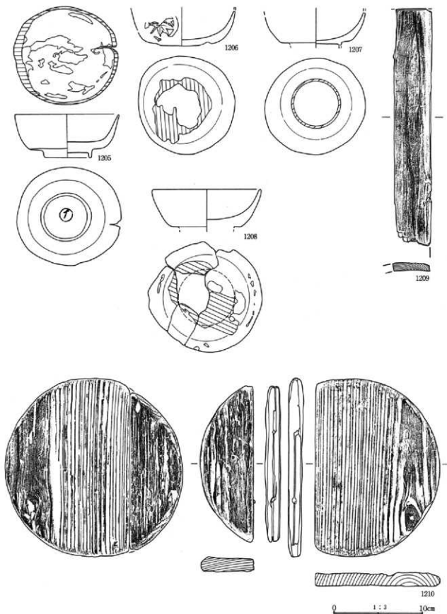
第224図 B区24号井戸出土木製品
