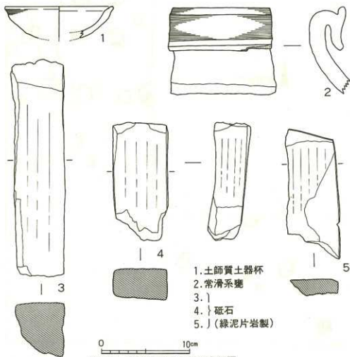
第8図 徳尾遺跡出土遺物実測図
